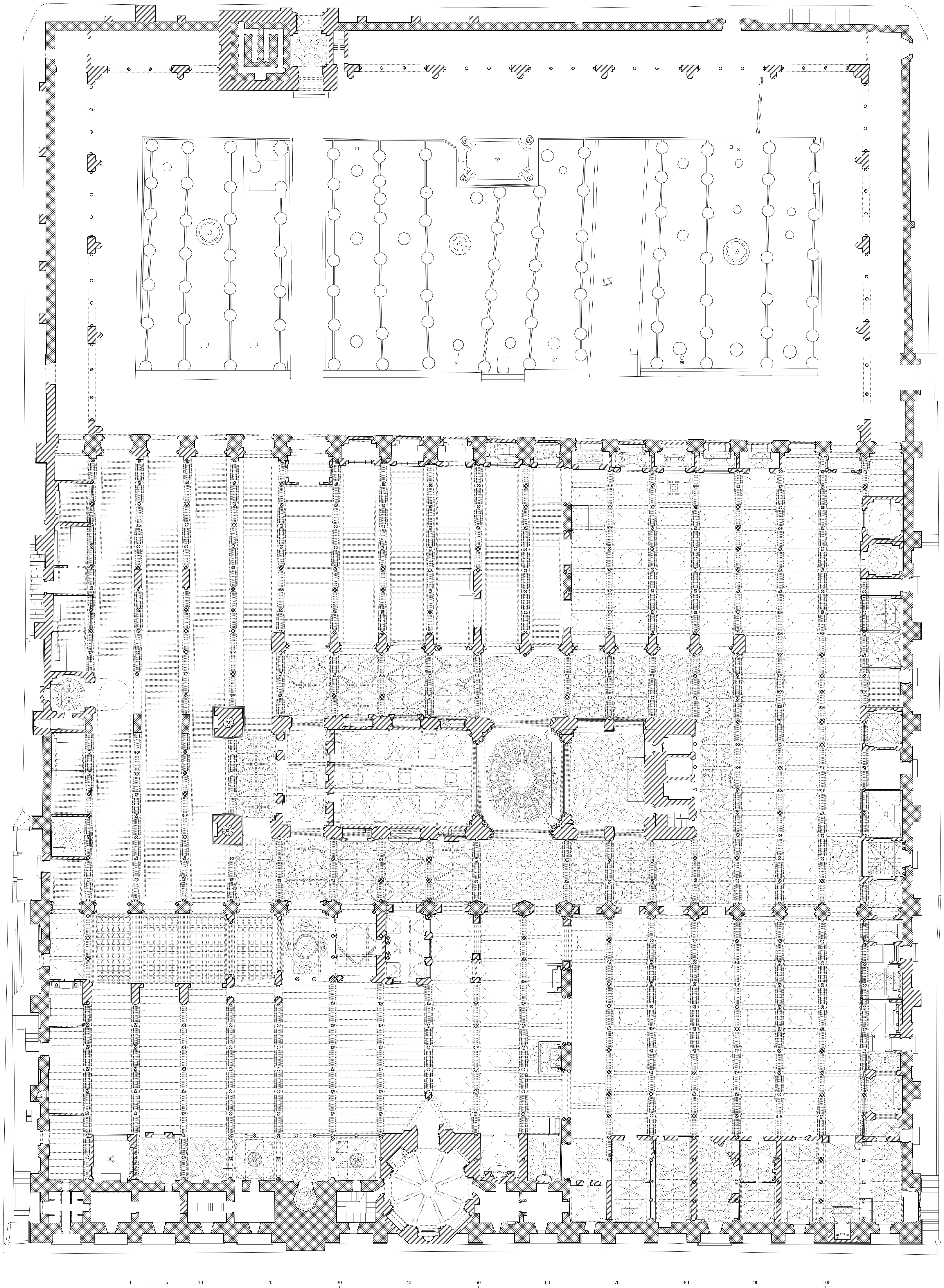
CATEDRAL EX-MEZQUITA DE CORDOBA. PLANTA. BASADO EN PLANOS DE F.HERNANDEZ (1930) Y K.A.C.CRESWELL (1940) - ESCUELA DE ESTUDIOS ARABES, C.S.I.C. A.ALMAGRO
