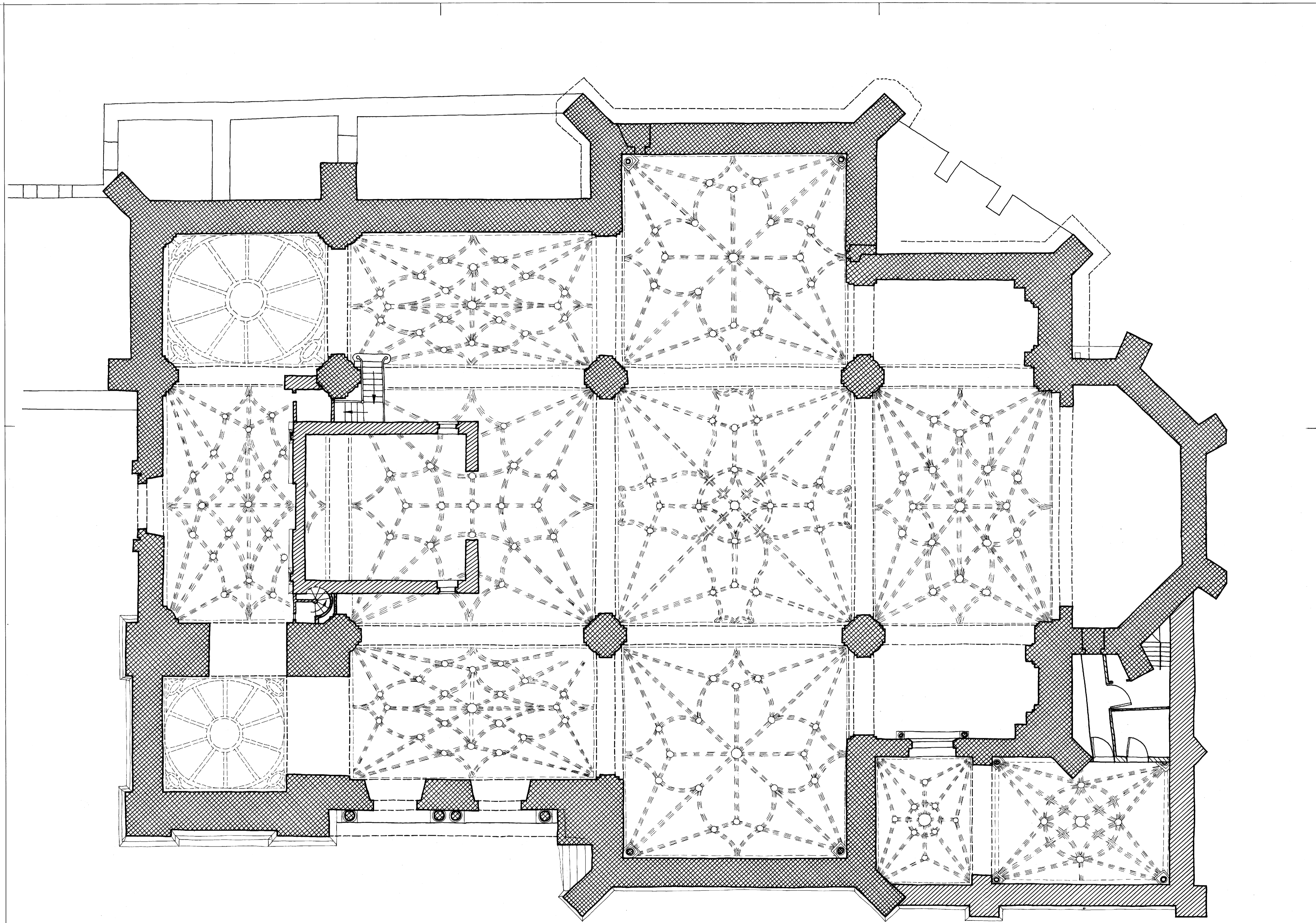
IGLESIA PARROQUIAL NAVARRETE (LOGROÑO) PLANTA E: 1/100 A. ALMAGRO / arq. JUNIO 1975
