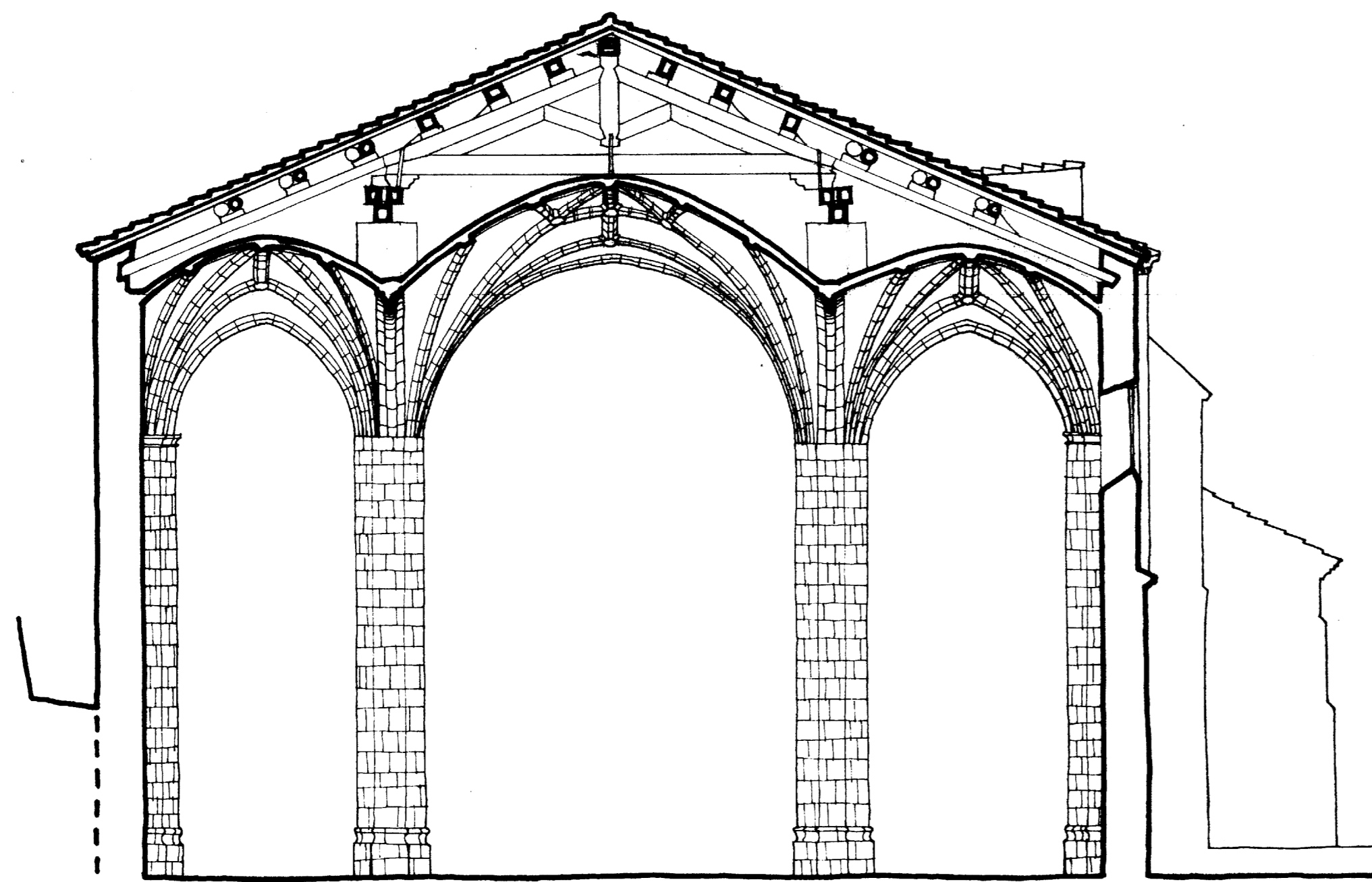
SECCION TRANSVERSAL
