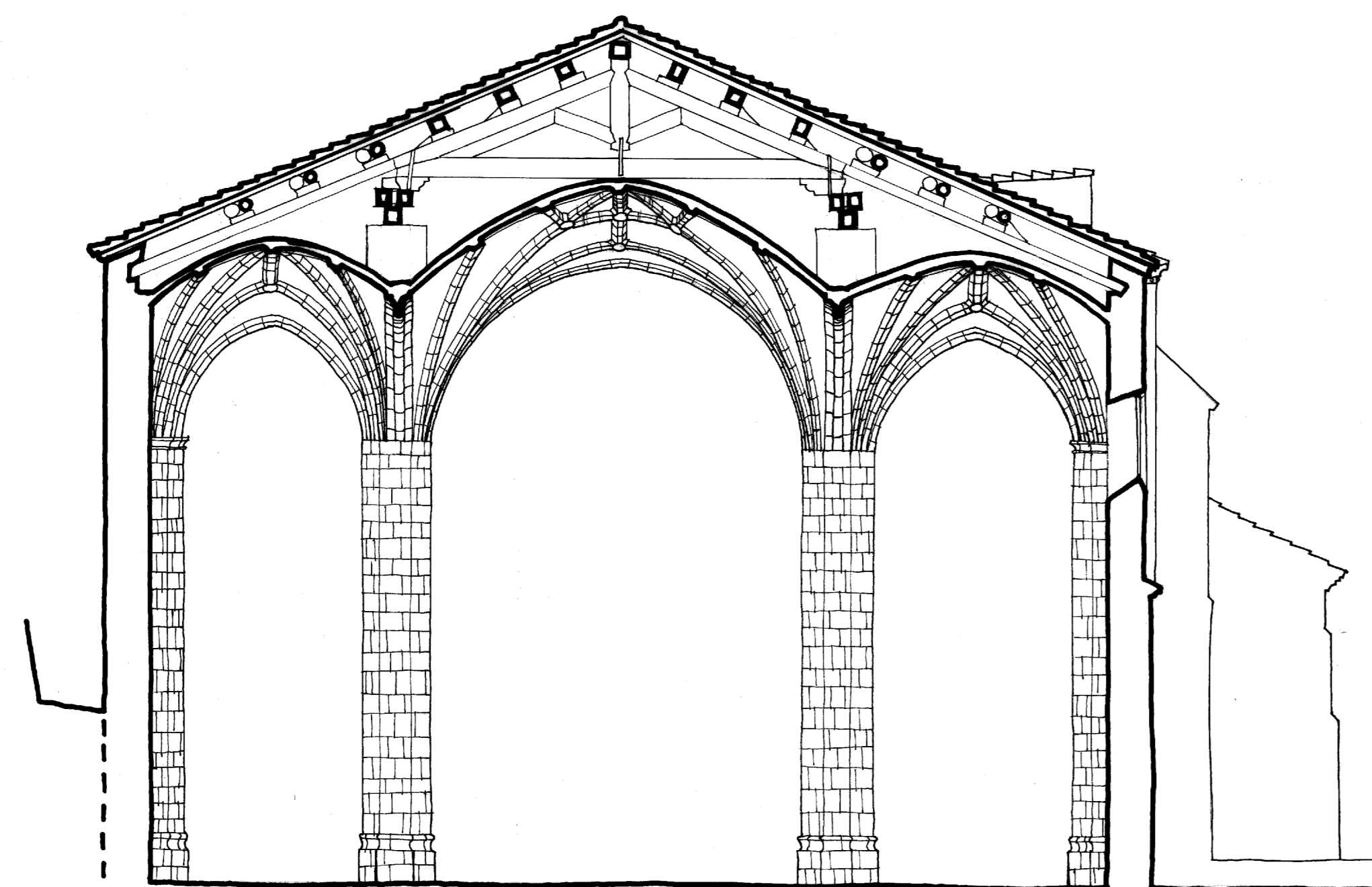
SECCION TRANSVERSAL
