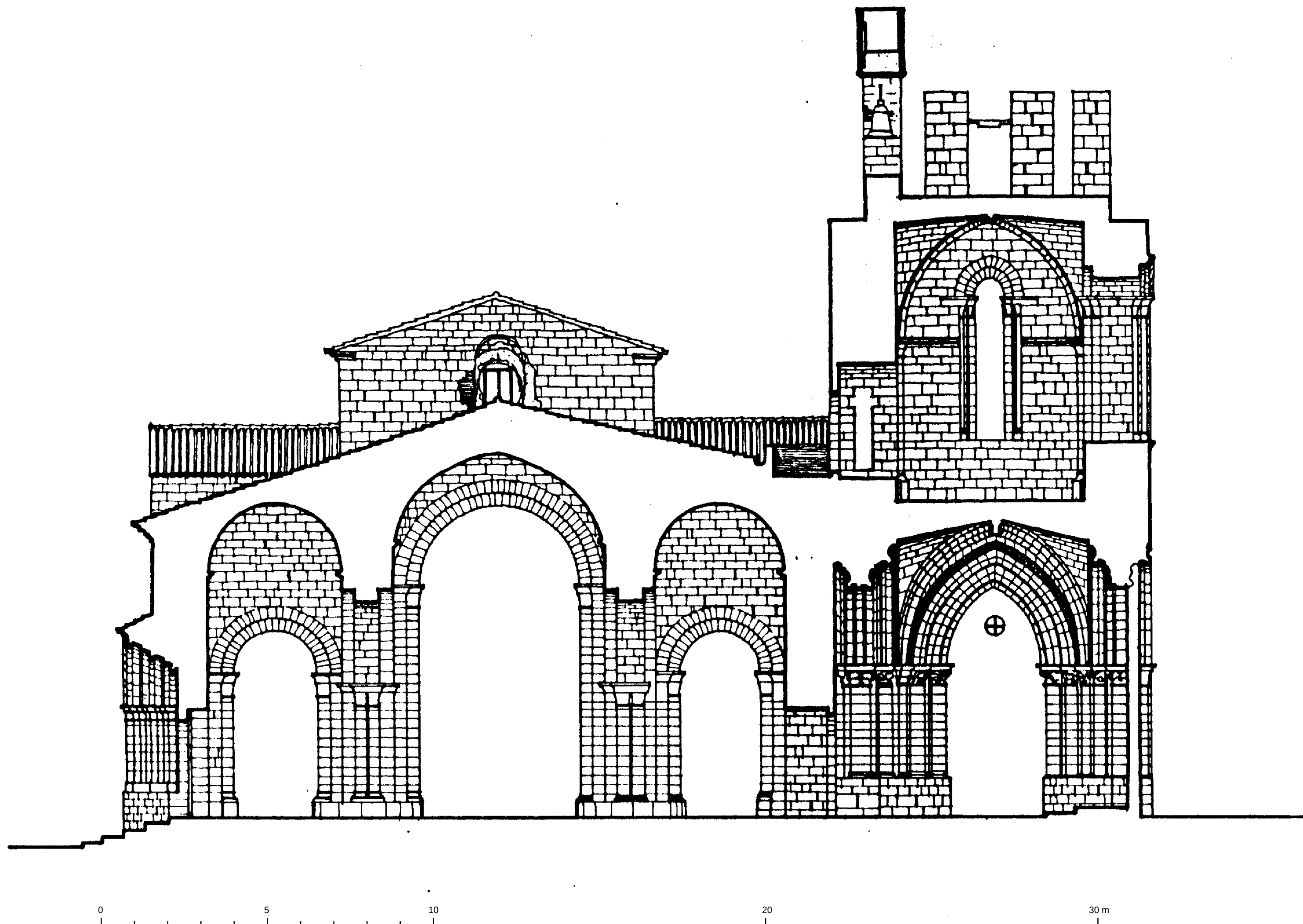
IGLESIA DE SANTA MARIA LA BLANCA, BERBEGAL (HUESCA). SECCION TRANSVERSAL, ESTADO INICIAL A. Almagro / arq. 1976
