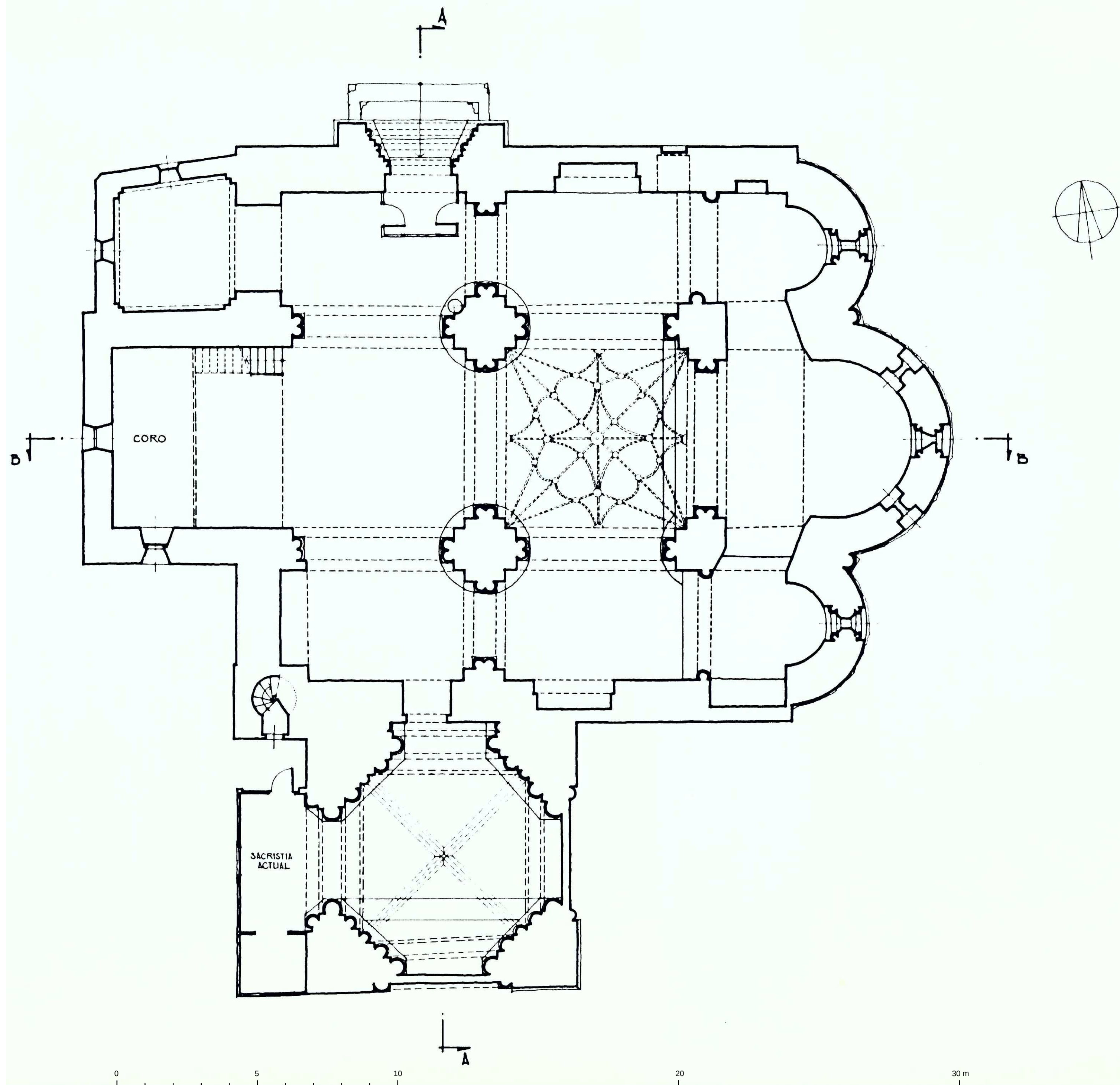
IGLESIA DE SANTA MARIA LA BLANCA, BERBEGAL (HUESCA). PLANTA ESTADO INICIAL A. Almagro / arq. 1976
