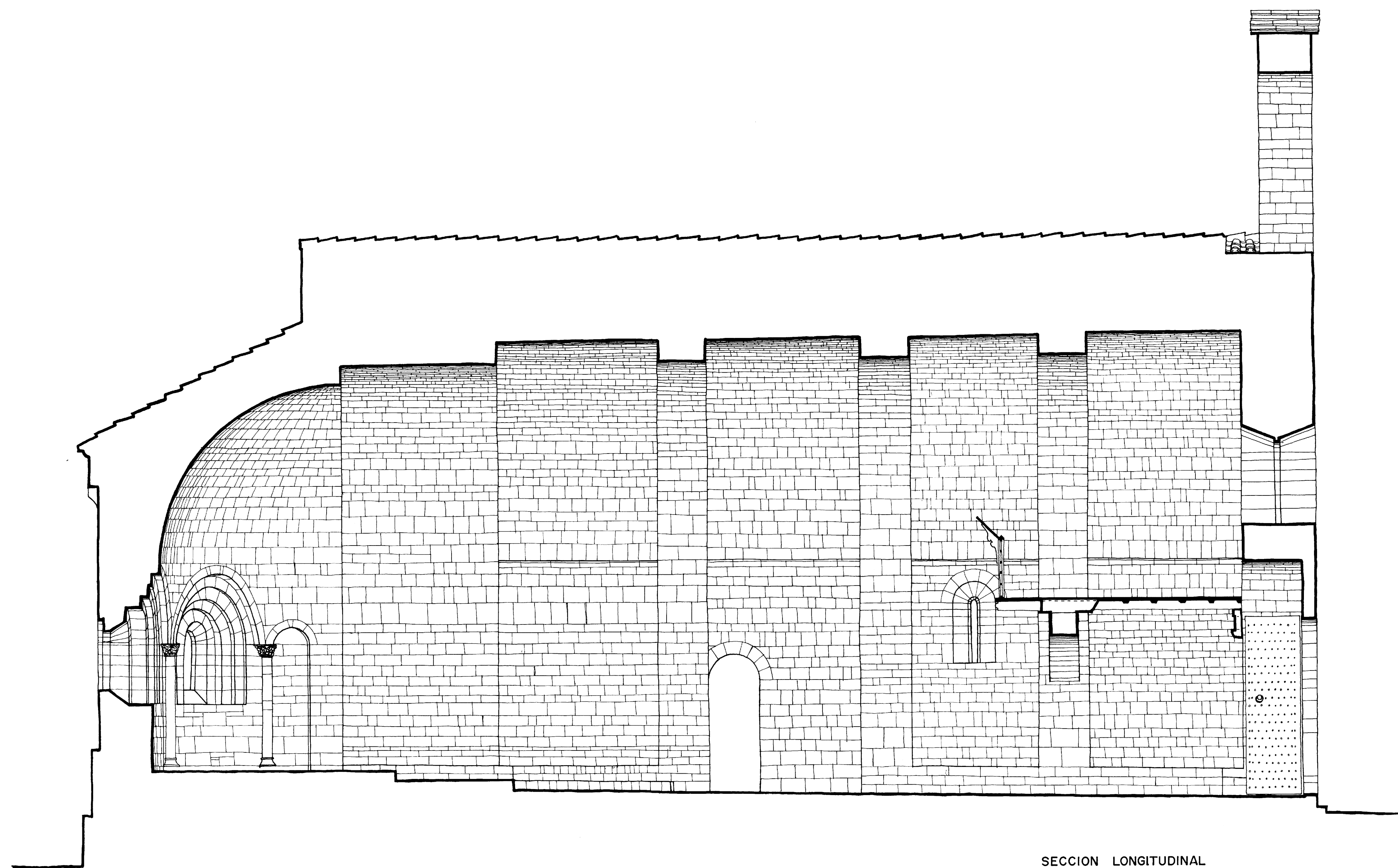
SECCION LONGITUDINAL
