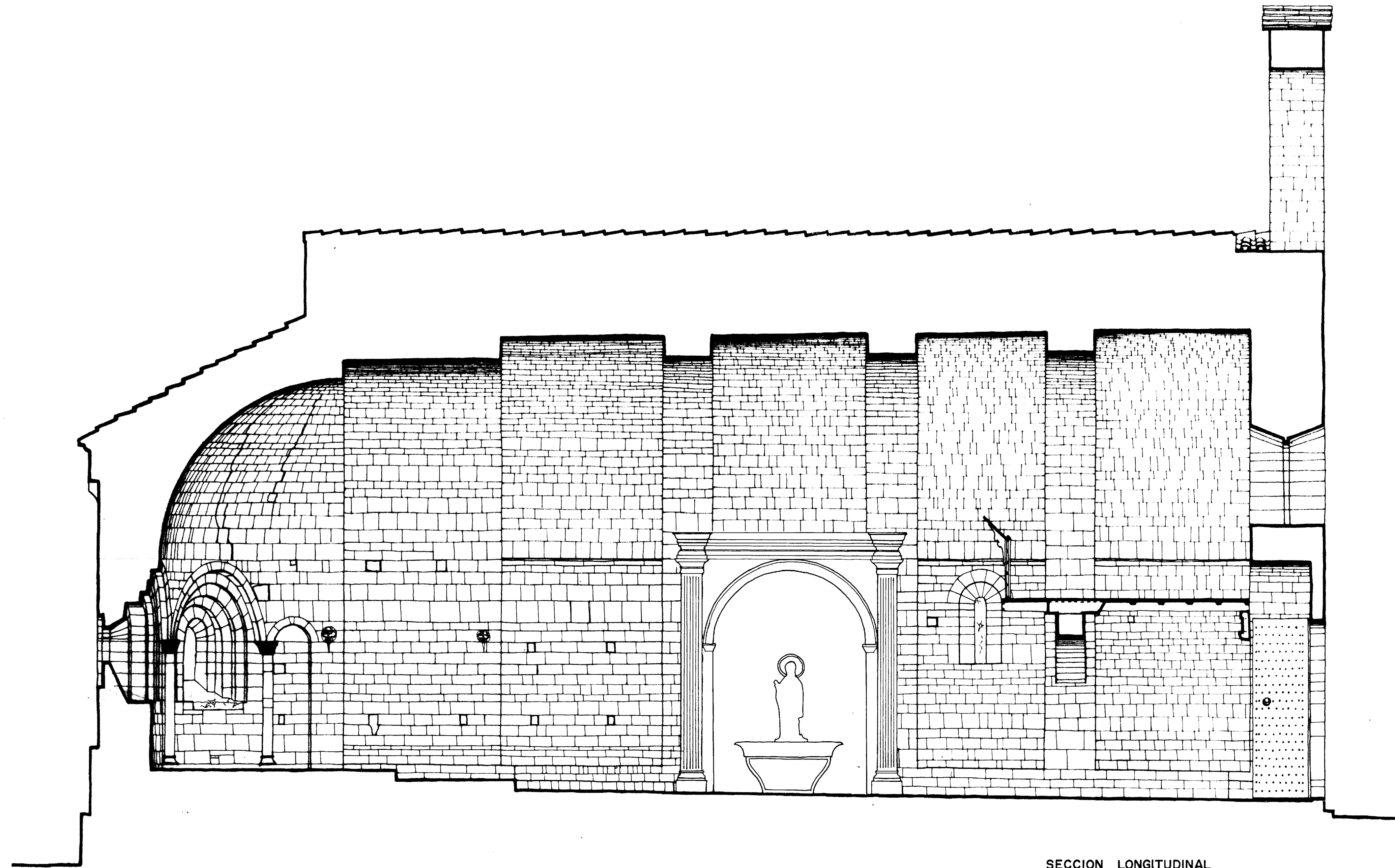
SECCION LONGITUDINAL
