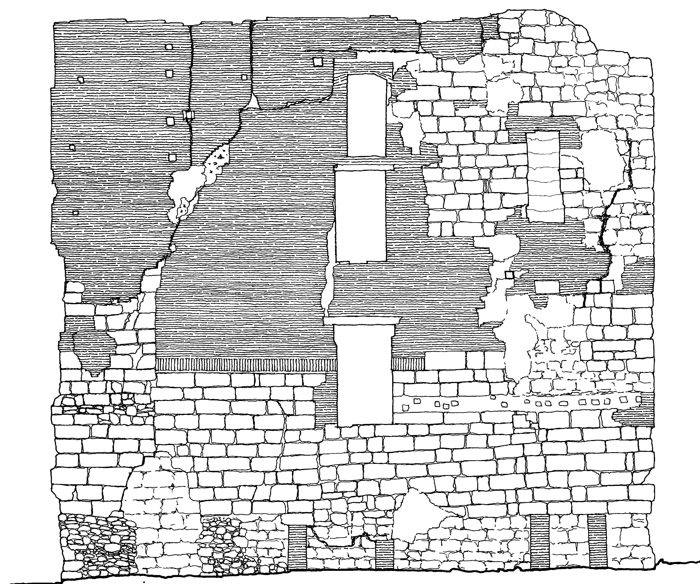
ALZADO SUR
