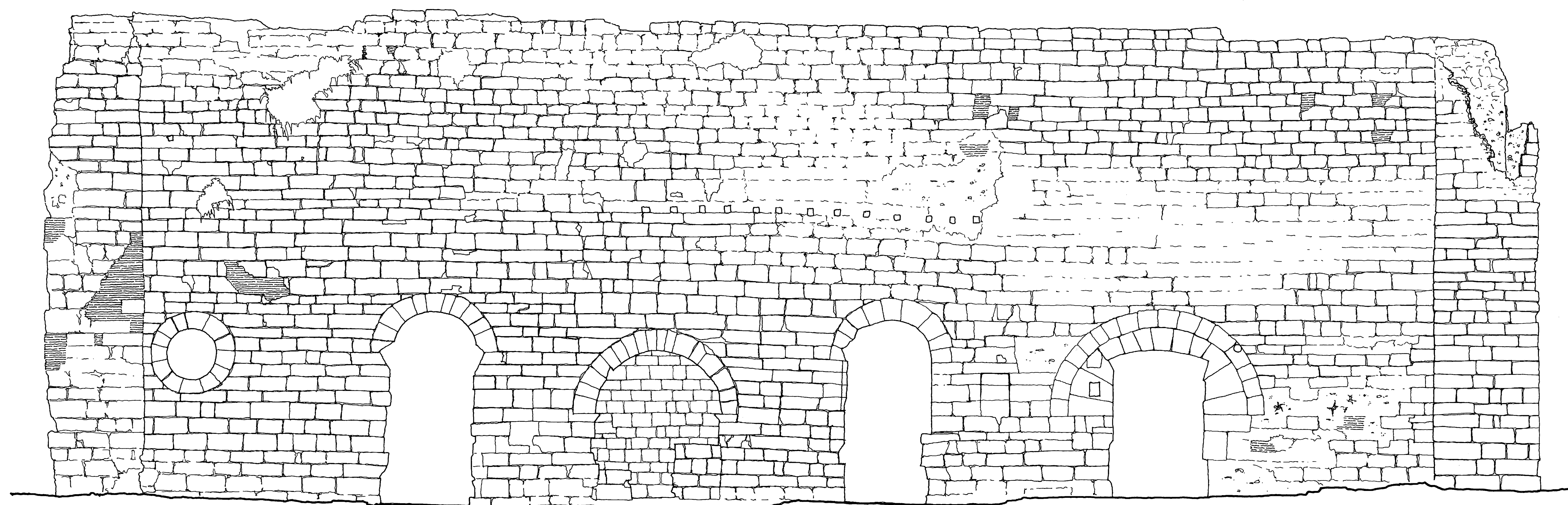
ALZADO ESTE
