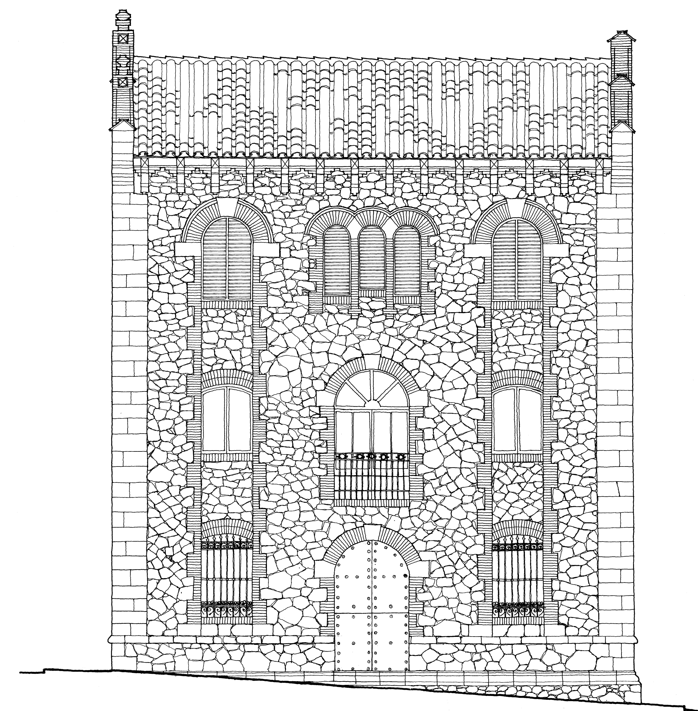
alzado lateral clerecía
