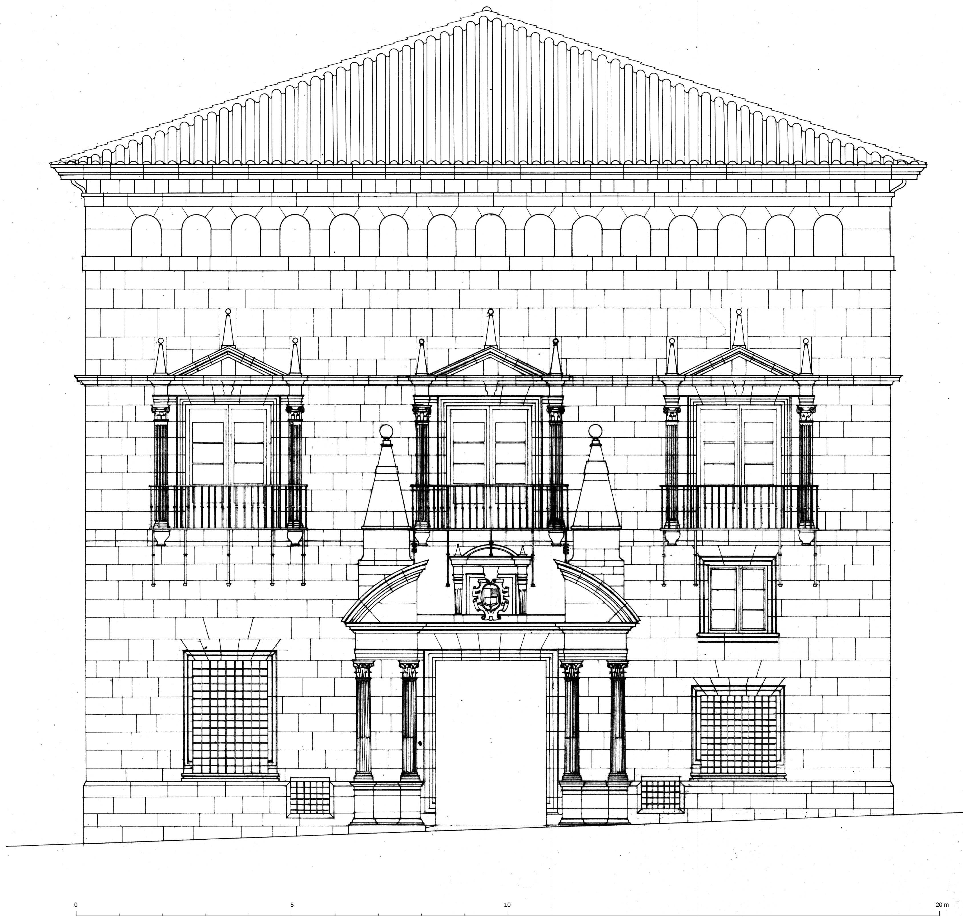
CASA DE LA COMUNIDAD DE TERUEL. HIPOTESIS DE SU TRAZADO ORIGINAL A. Almagro / arq.
