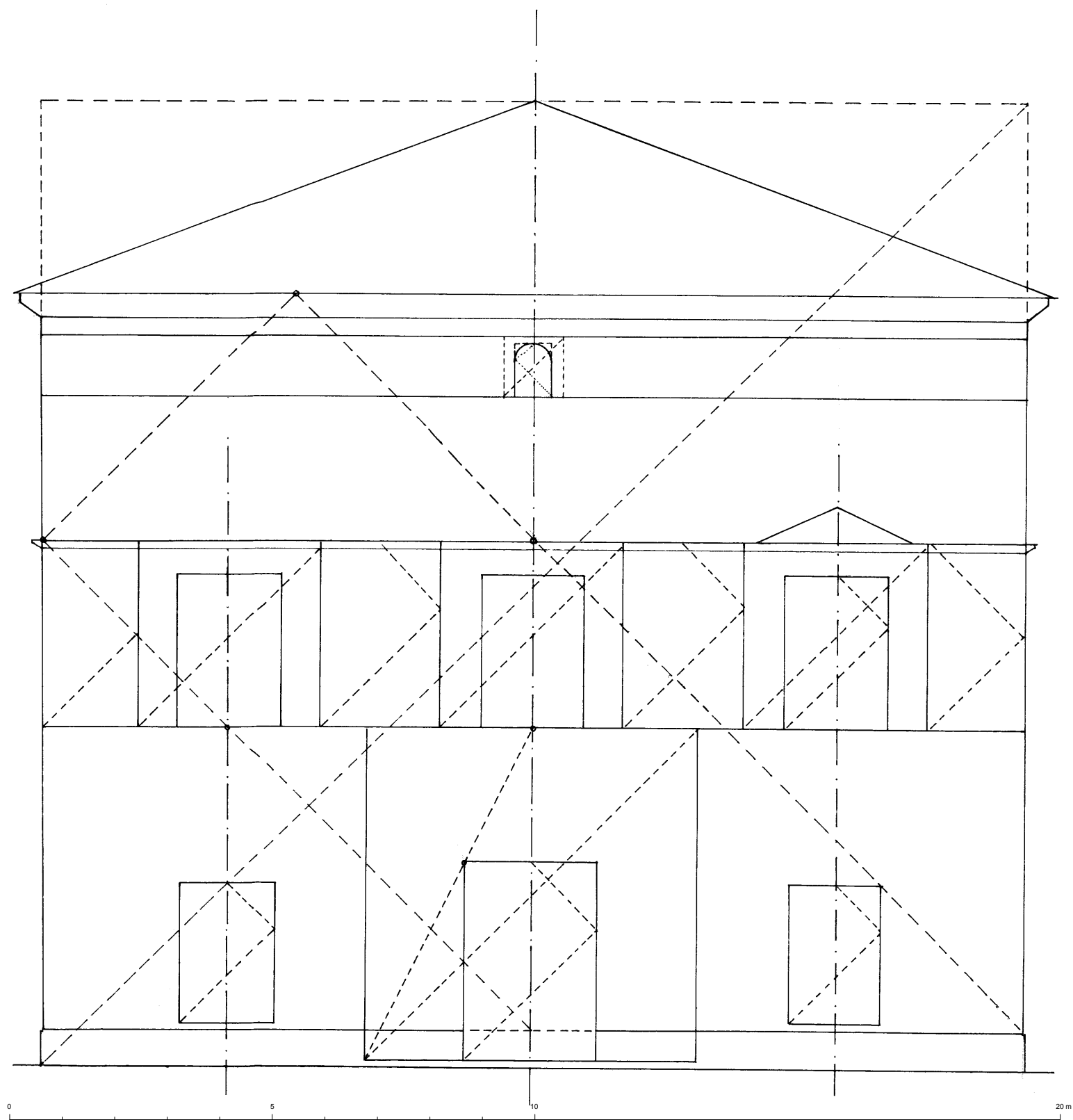
CASA DE LA COMUNIDAD DE TERUEL. HIPOTESIS DE SU TRAZADO GEOMETRICO A. Almagro / arq.
