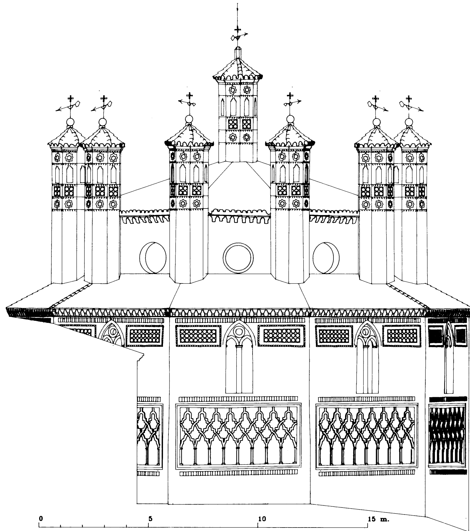
IGLESIA DE SAN PEDRO DE TERUEL. ALZADO CABECERA
