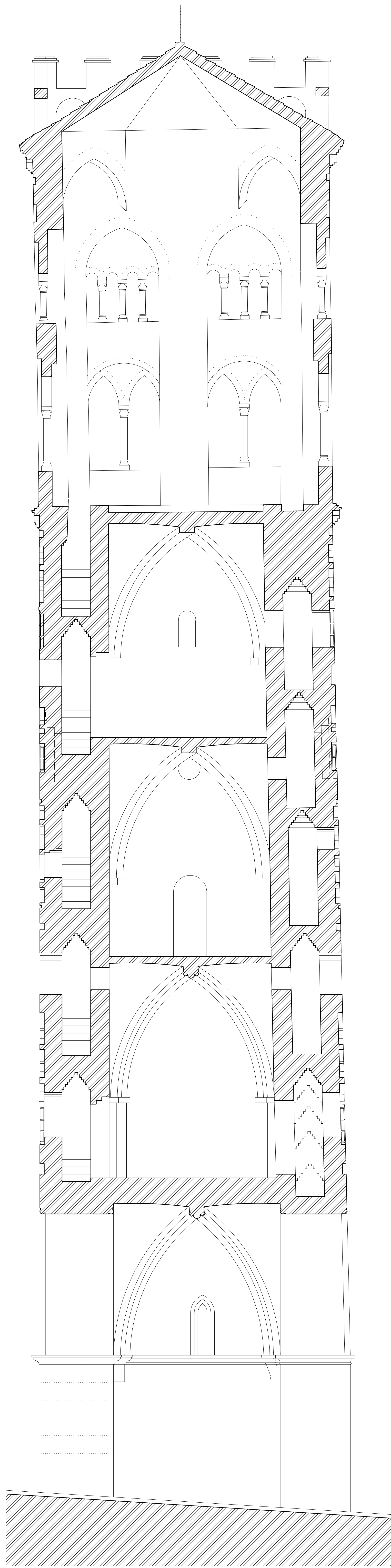
IGLESIA DEL SALVADOR DE TERUEL. SECCION DE LA TORRE. A. Almagro / arq. 1990
