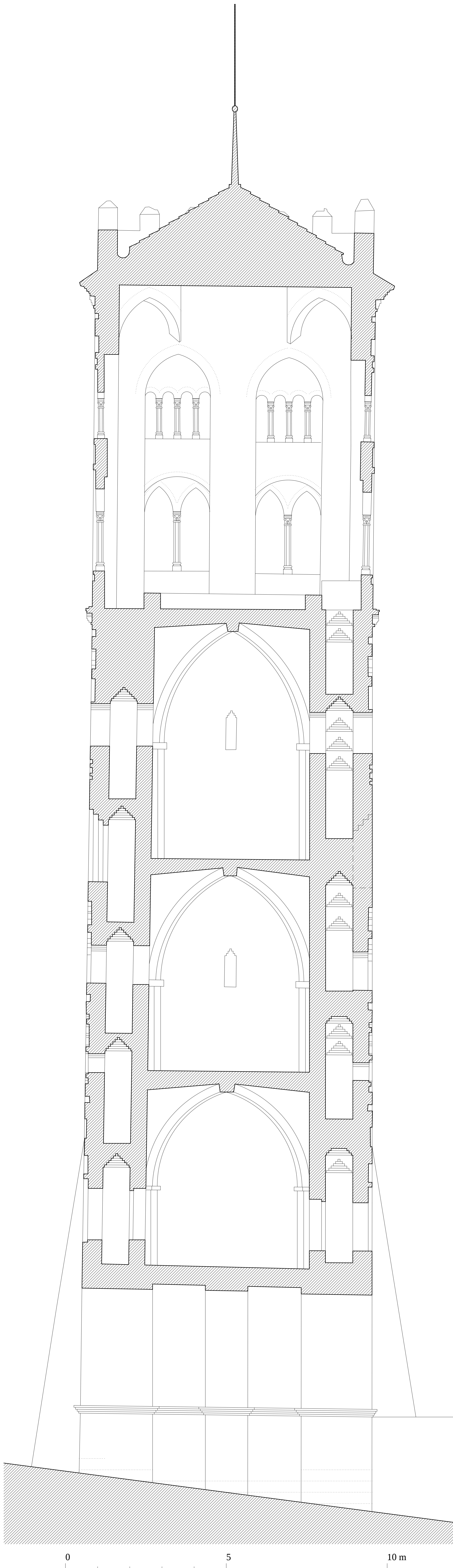
IGLESIA DE SAN MARTIN DE TERUEL. SECCION DE LA TORRE POR EL EJE. A. Almagro / arq. 1990
