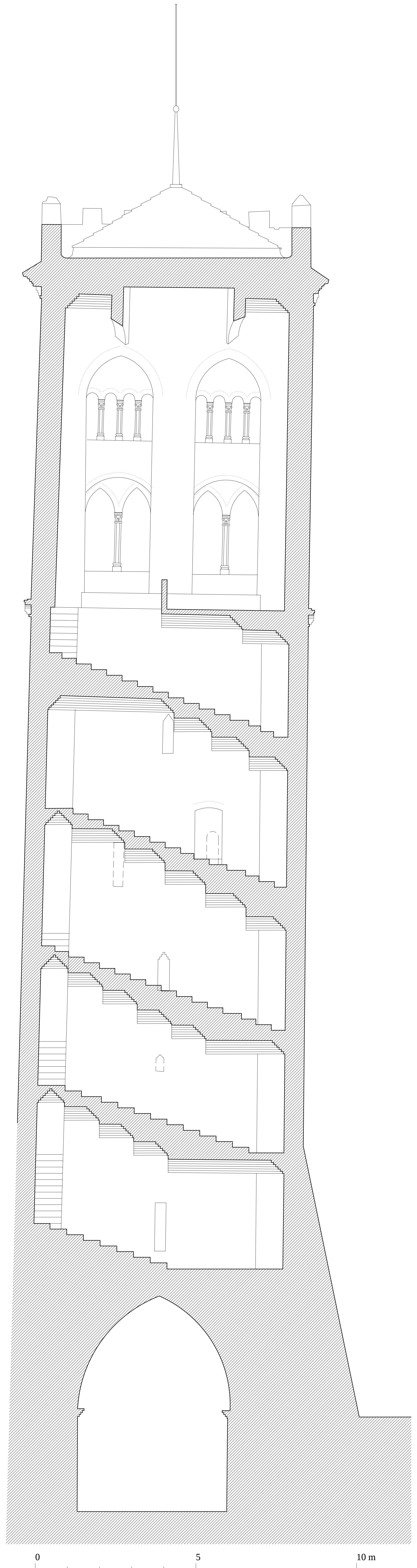
IGLESIA DE SAN MARTIN DE TERUEL. SECCION DE LA TORRE POR LA ESCALERA. A. Almagro / arq. 1990
