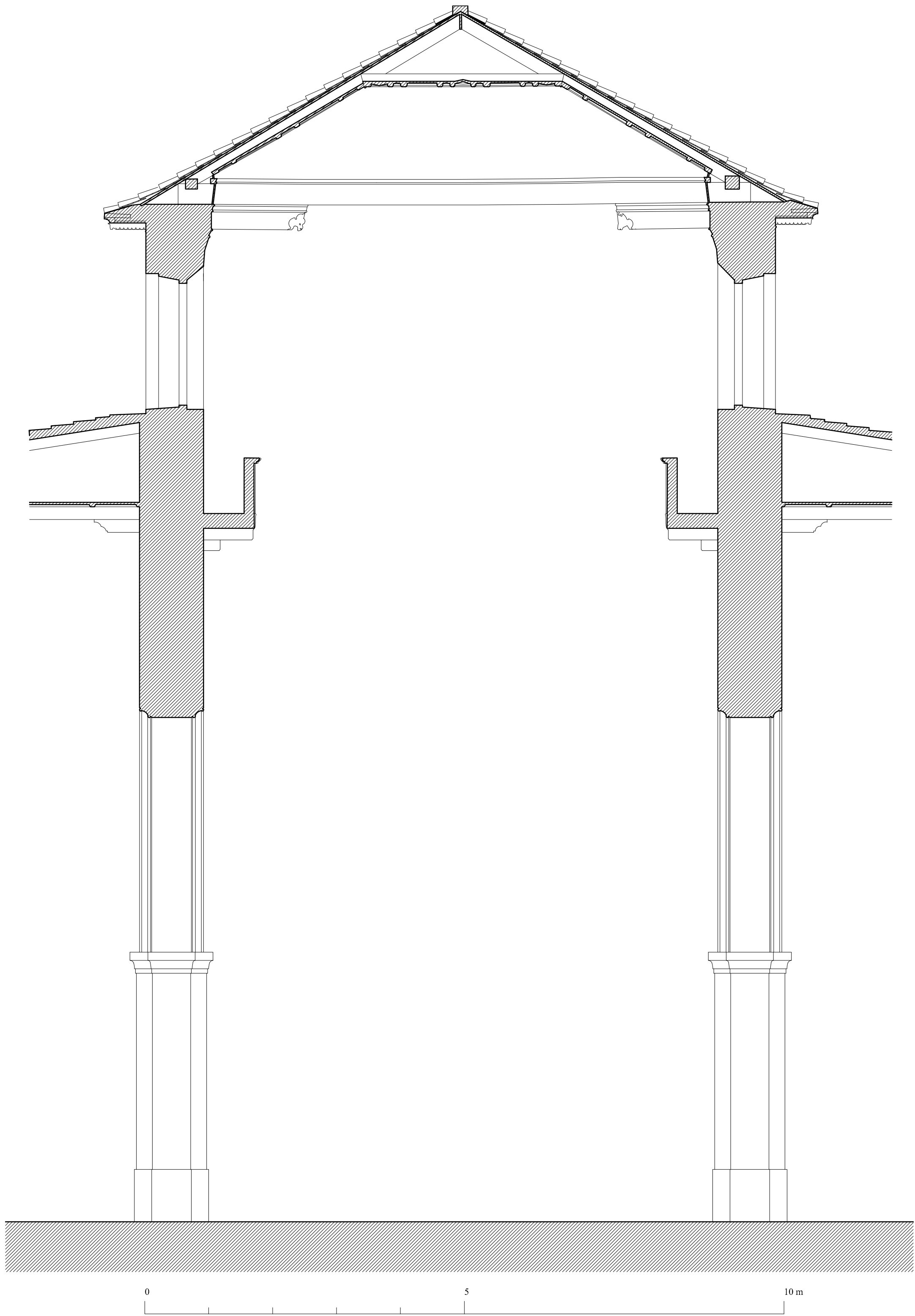
CATEDRAL DE TERUEL. SECCION TRANSVERSAL DE LA NAVE. A. Almagro / arq. 1990
