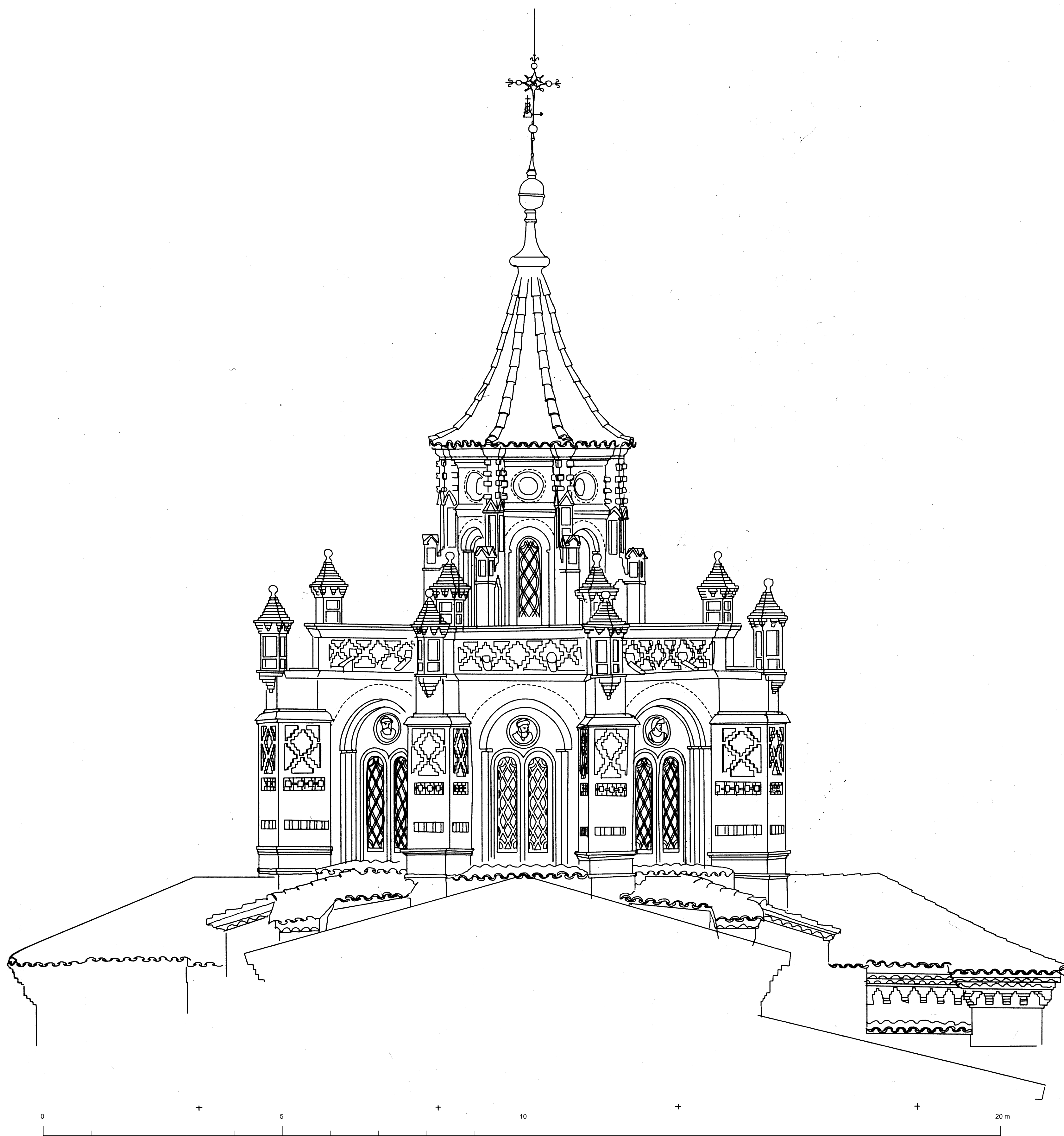
CATEDRAL DE TERUEL. ALZADO EXTERIOR NORTE DEL CIMBORRIO. A. Almagro / arq. 1990
