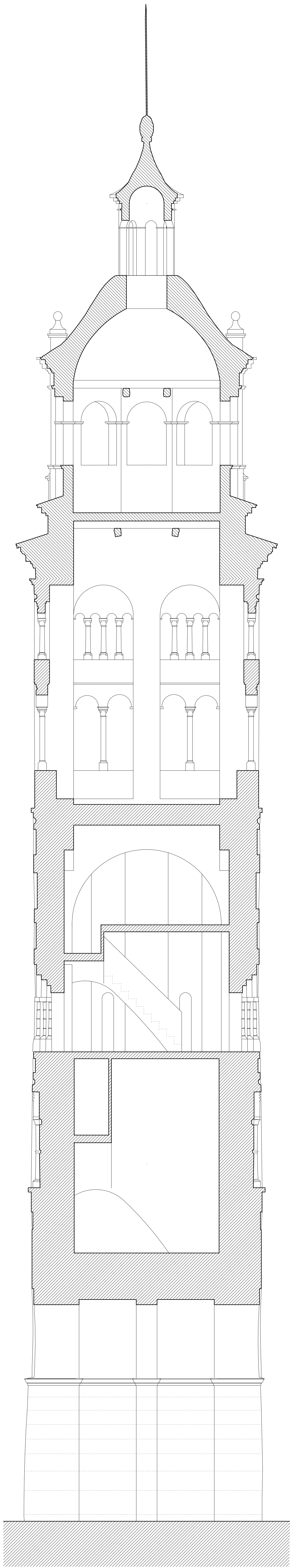
0 5 m CATEDRAL DE TERUEL. SECCIÓN DE LA TORRE. A. Almagro / arq. 1990
