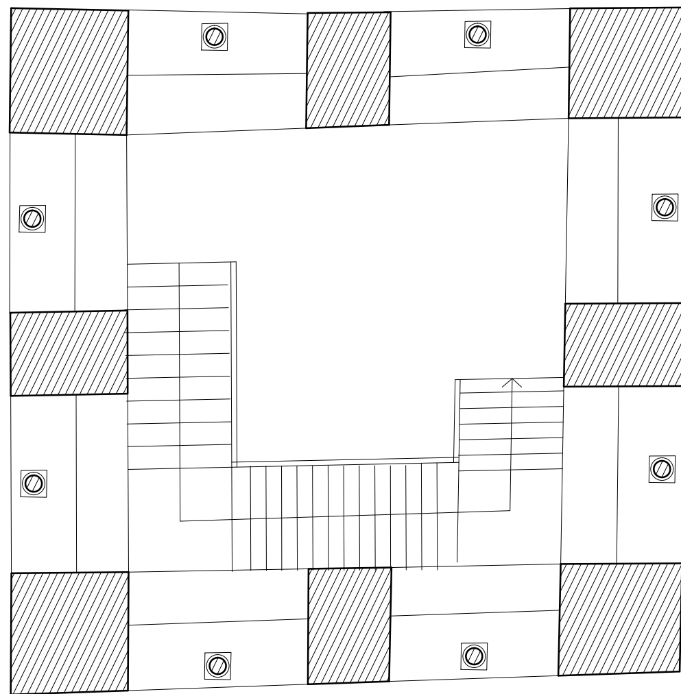
0 5 m CATEDRAL DE TERUEL. PLANTA 4 DE LA TORRE. A. Almagro / arq. 1990
