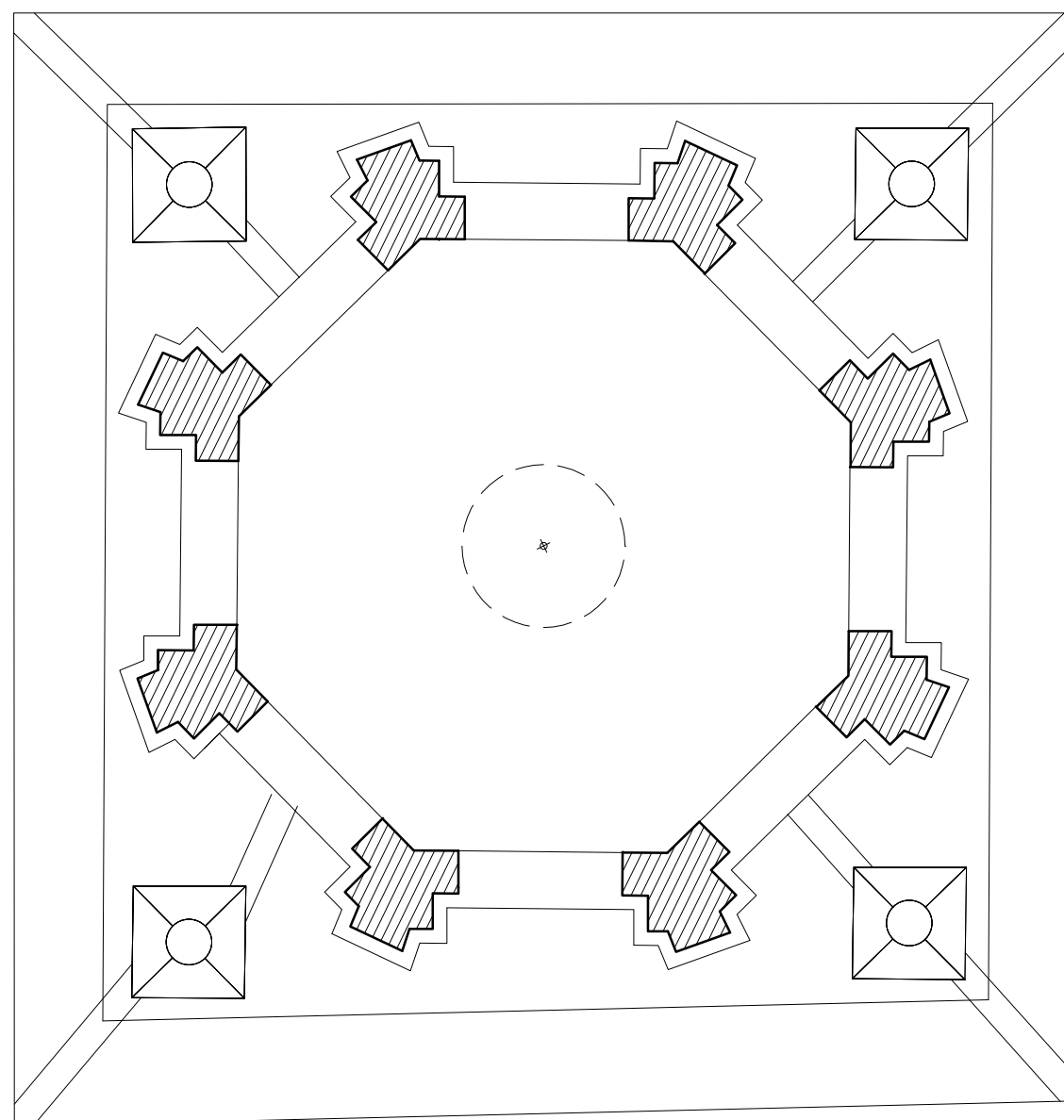
0 5 m CATEDRAL DE TERUEL. PLANTA 5 DE LA TORRE. A. Almagro / arq. 1990
