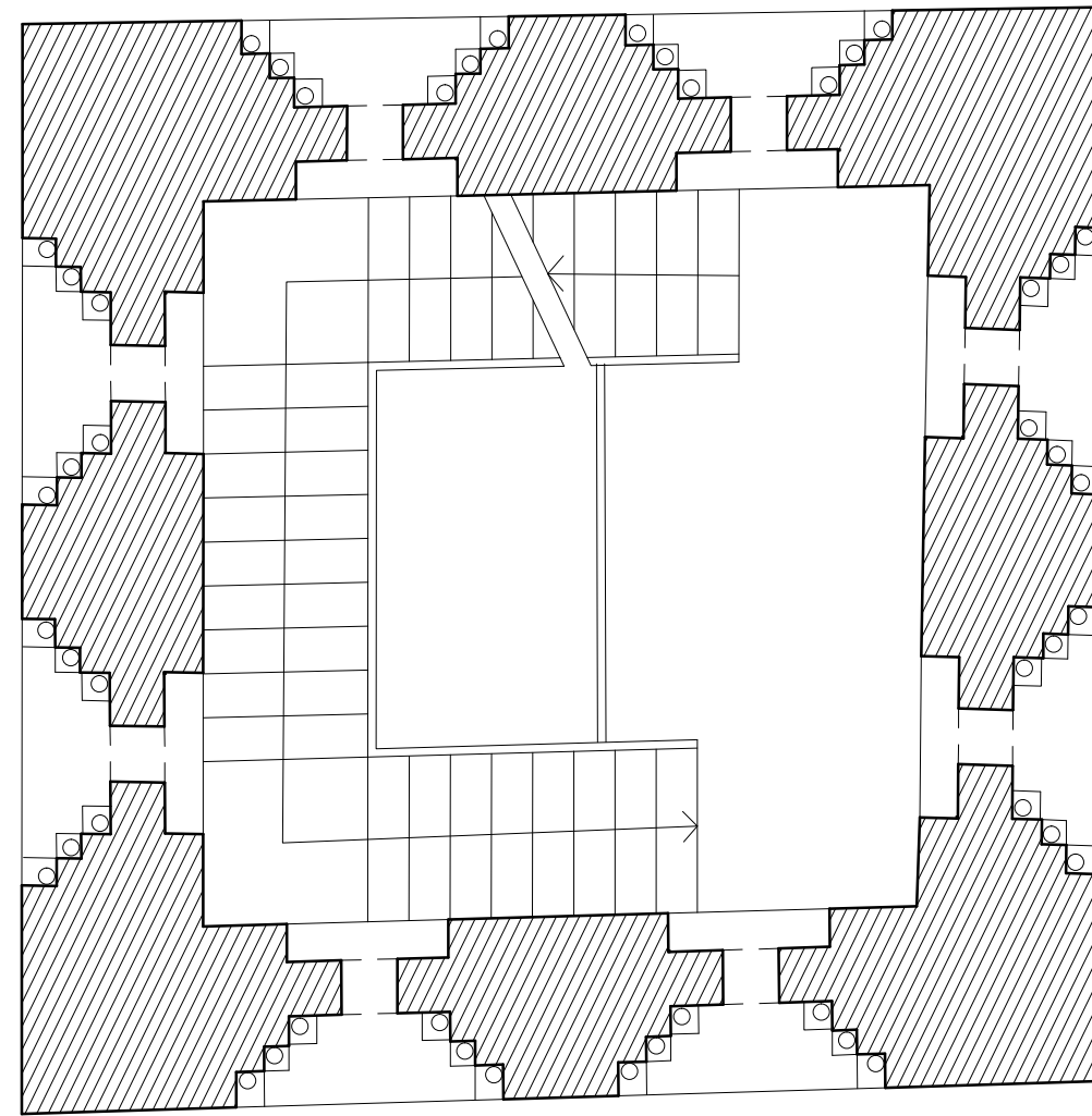
0 5 m CATEDRAL DE TERUEL. PLANTA 2 DE LA TORRE. A. Almagro / arq. 1990
