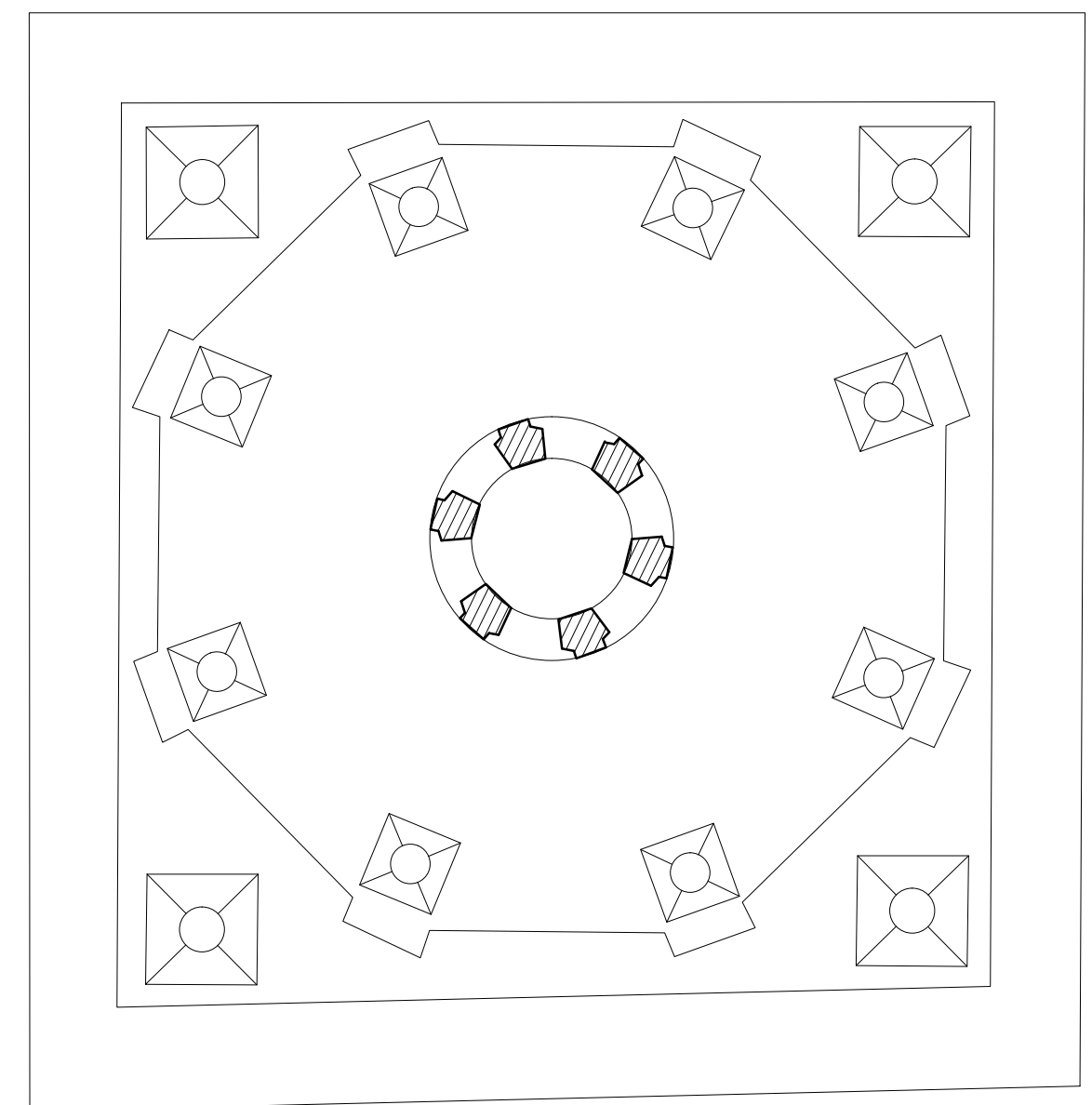
0 5 m CATEDRAL DE TERUEL. PLANTA 6 DE LA TORRE. A. Almagro / arq. 1990
