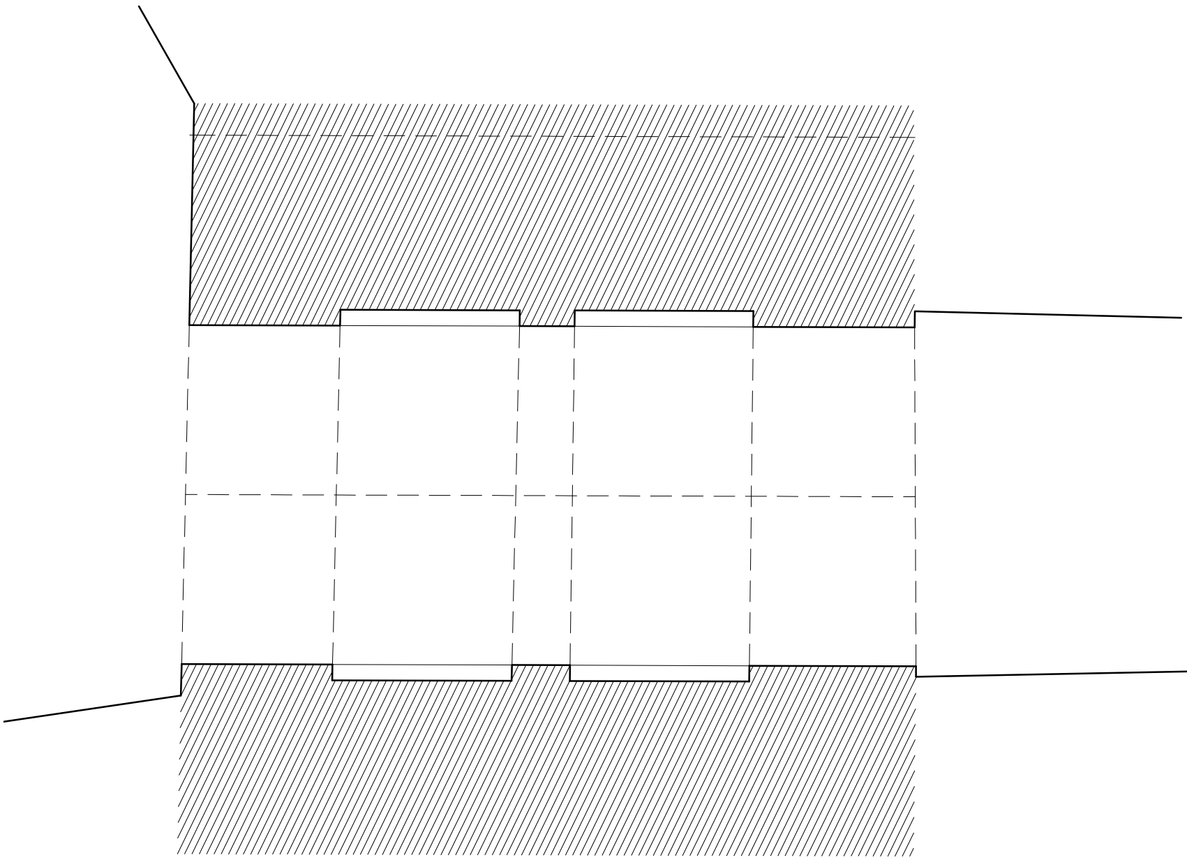
0 5 m CATEDRAL DE TERUEL. PLANTA 1 DE LA TORRE. A. Almagro / arq. 1990
