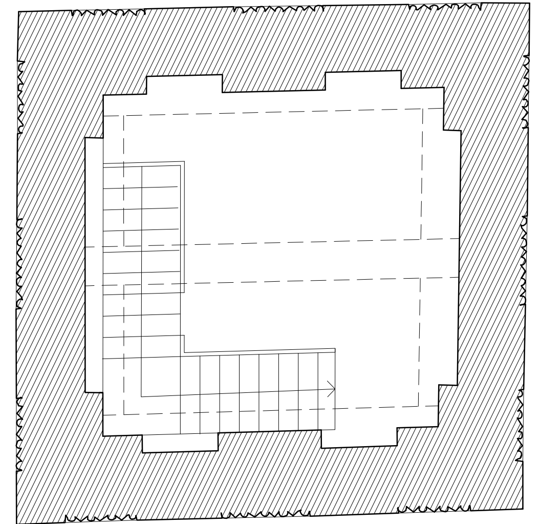
0 5 m CATEDRAL DE TERUEL. PLANTA 3 DE LA TORRE. A. Almagro / arq. 1990
