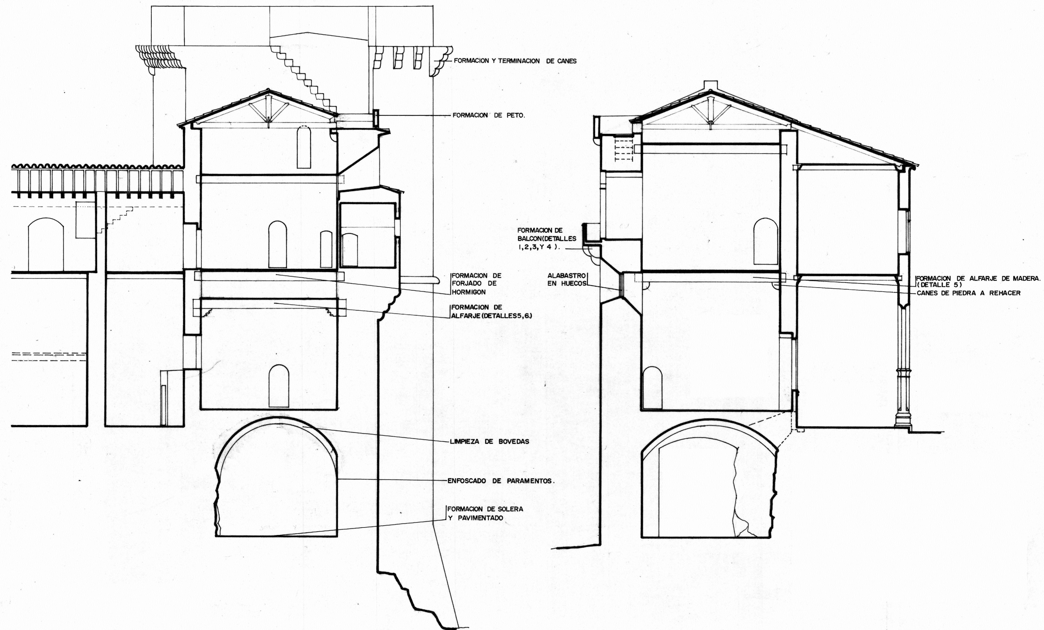
SECCION K-L
