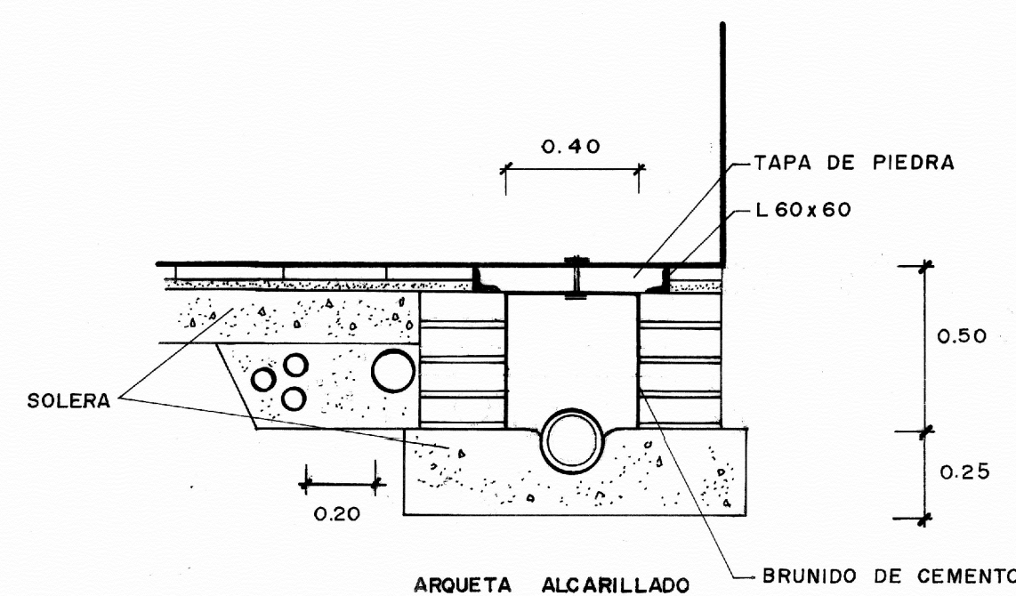
DETALLE I
