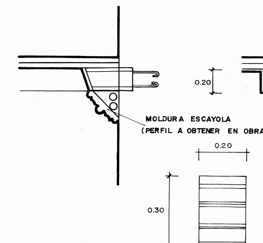
DETALLE 9
