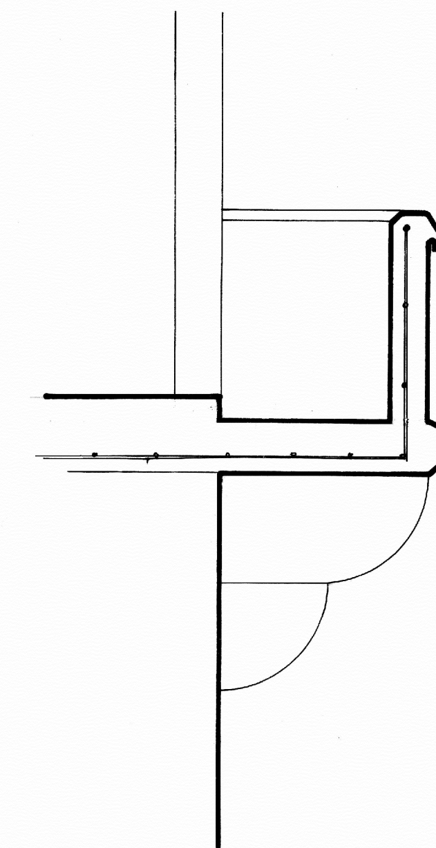
DETALLE 6
