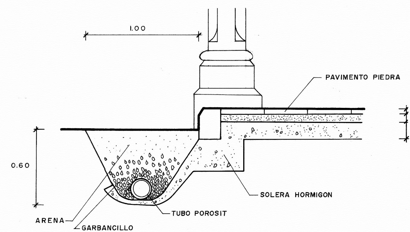
DETALLE O
