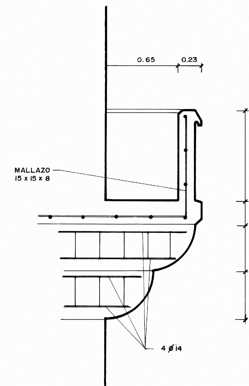
DETALLE 5
