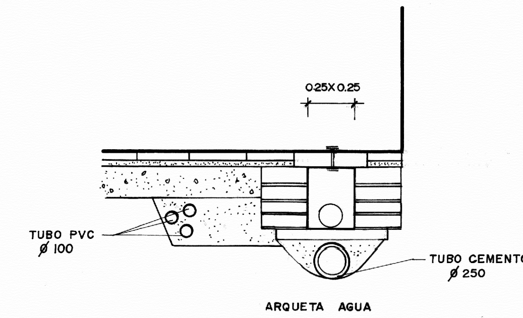
DETALLE 2
