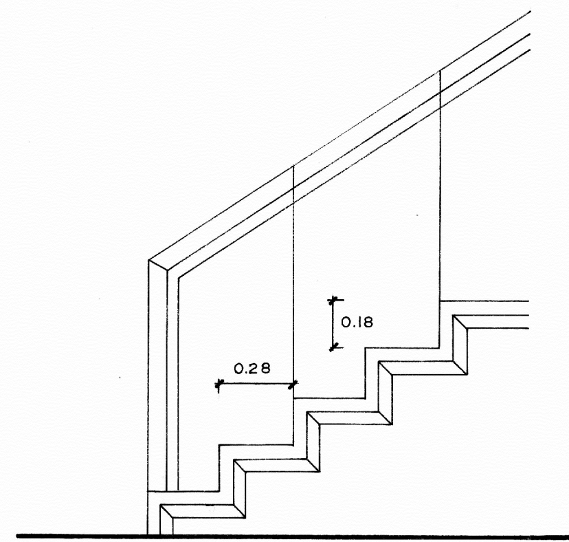
DETALLE 4
