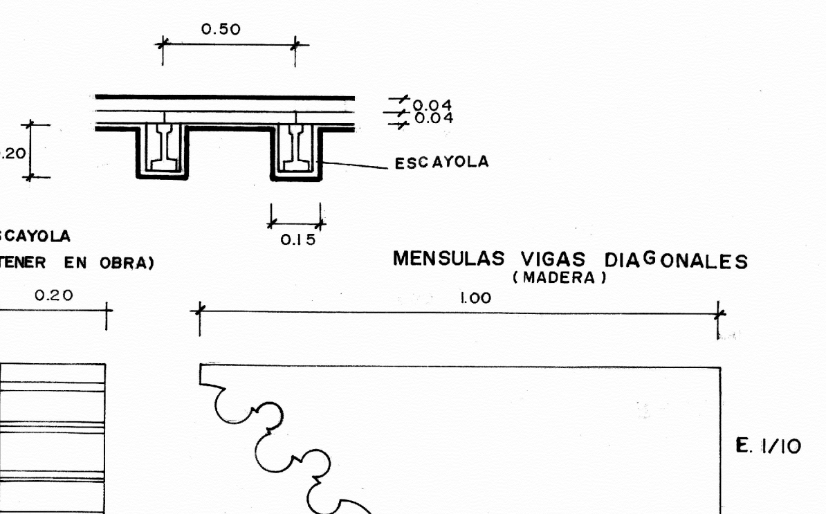
DETALLE 10
