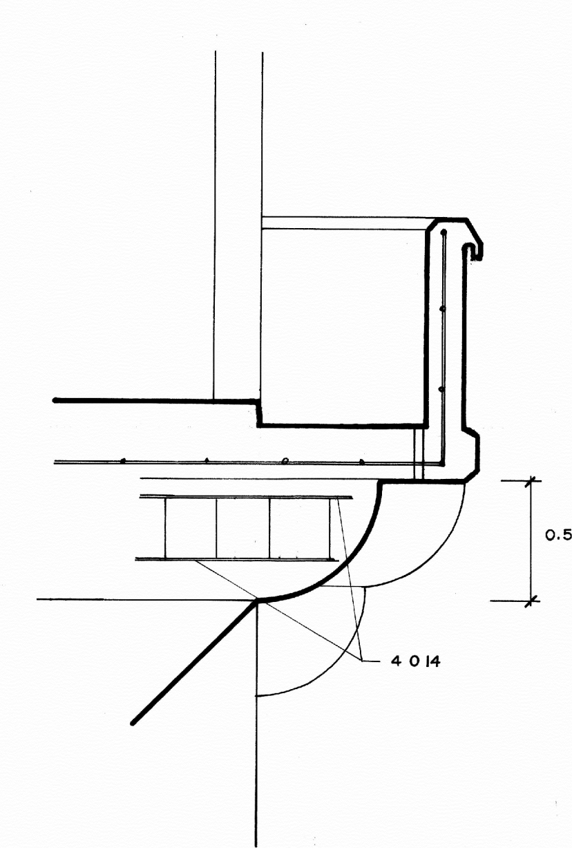
DETALLE 7
