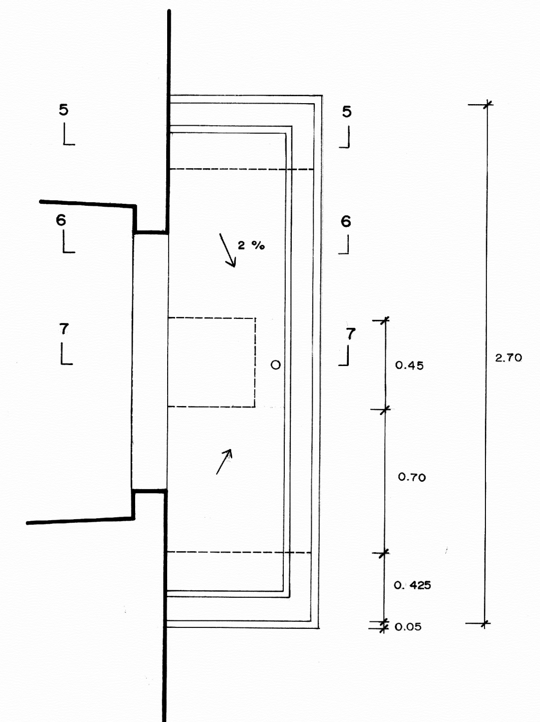
DETALLE 8
