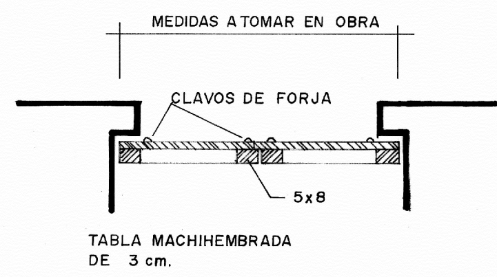
DETALLE PUERTAS
