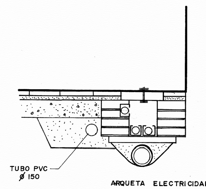
DETALLE 2'
