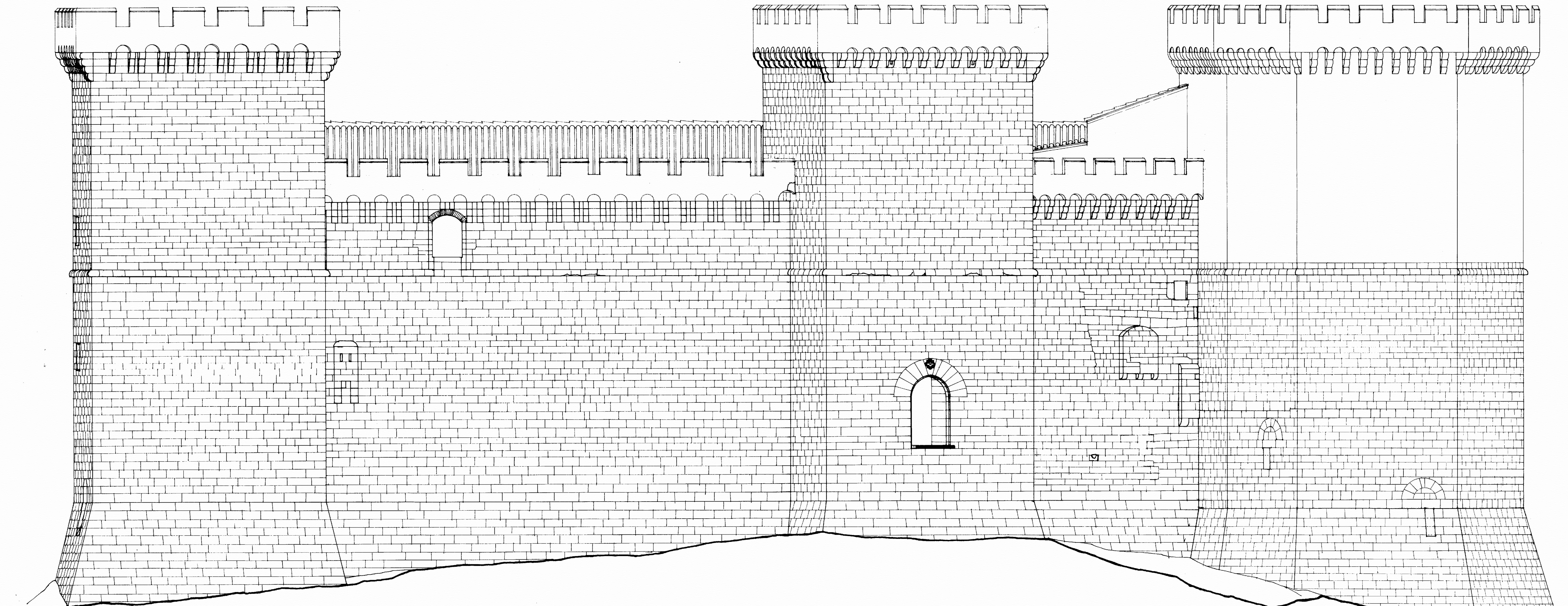
ALZADO N.E.
