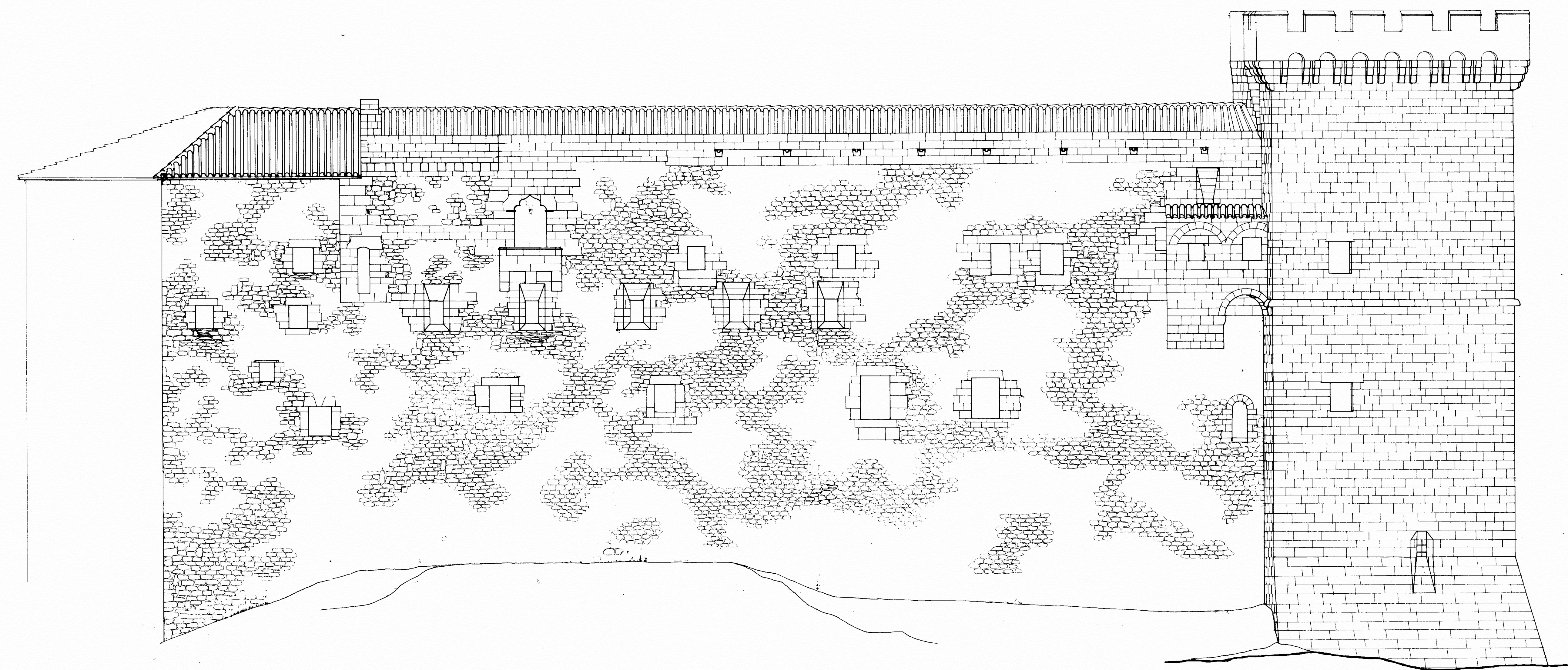
ALZADO S.E.
