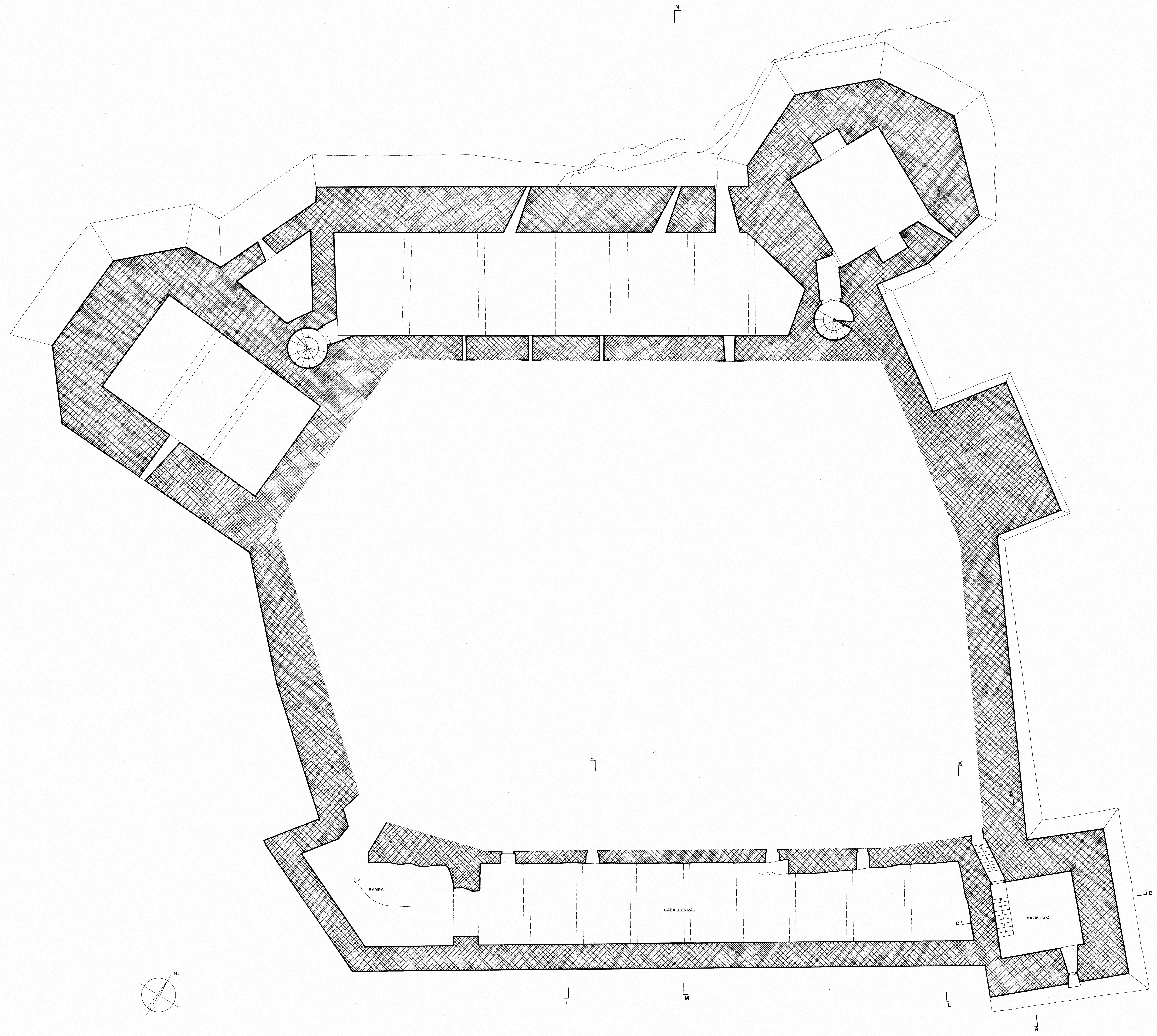
CASTILLO-PALACIO DE LOS FERNÁNDEZ DE HEREDIA EN MORA (TERUEL). SOTANOS. RESTAURACION. E. VIOO. F. PONCE DE LEÓN/ARG. AGOSTO 1984.
