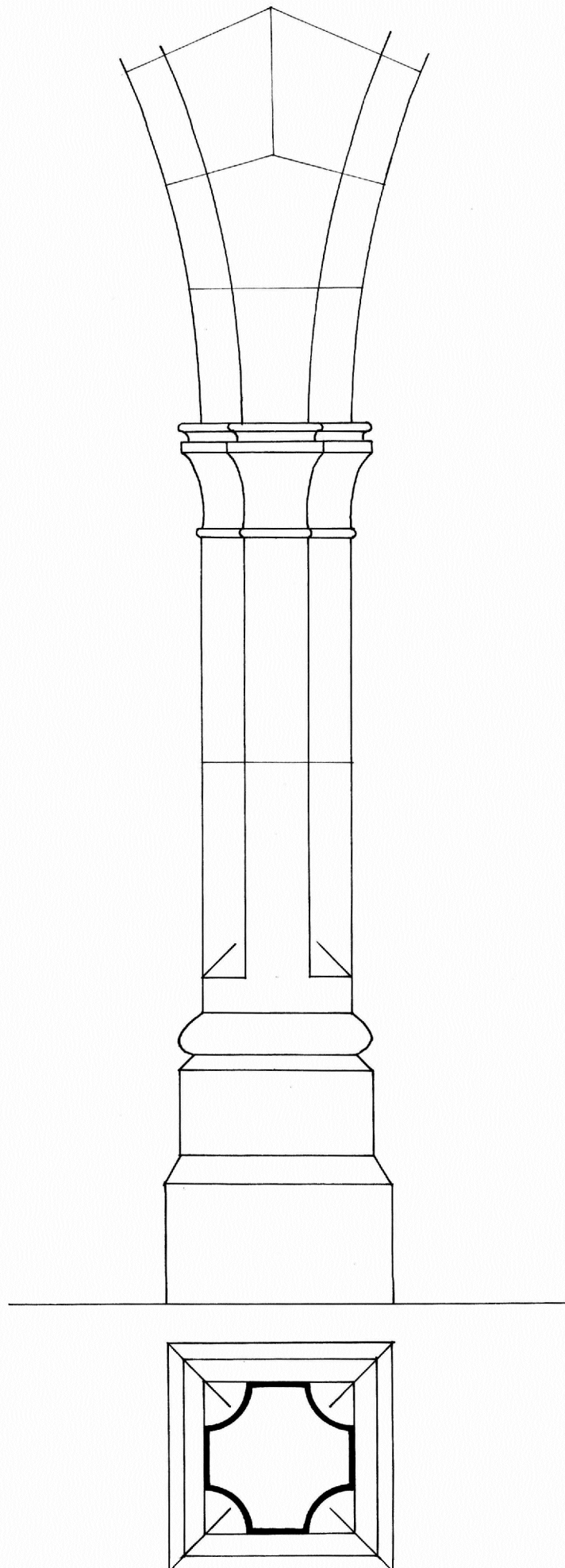
CASTILLO DE MORA ARQUERIA BAJA DEL PATIO. PILASTRA E. 1/20
