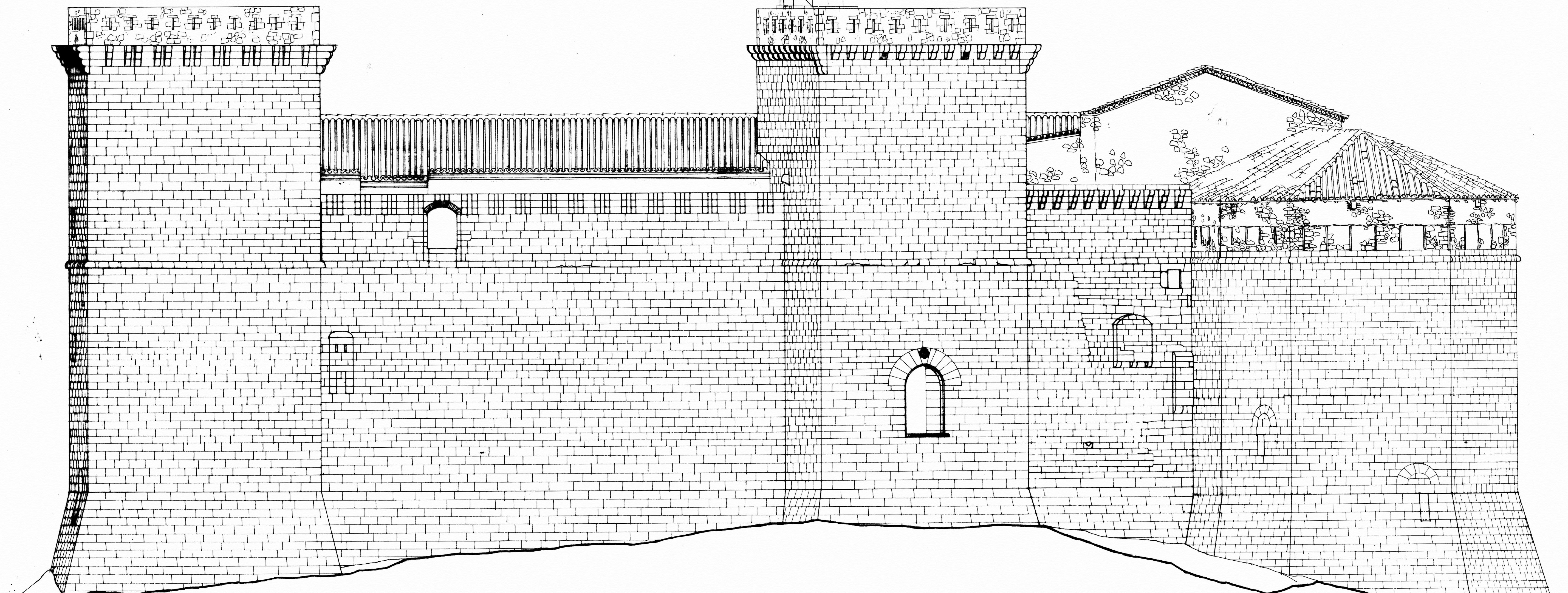
ALZADO N.E.
