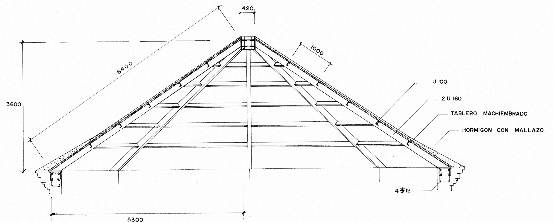
SECCION AB
