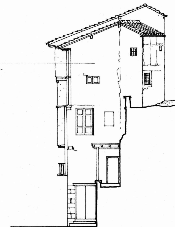
ALZADO LATERAL
