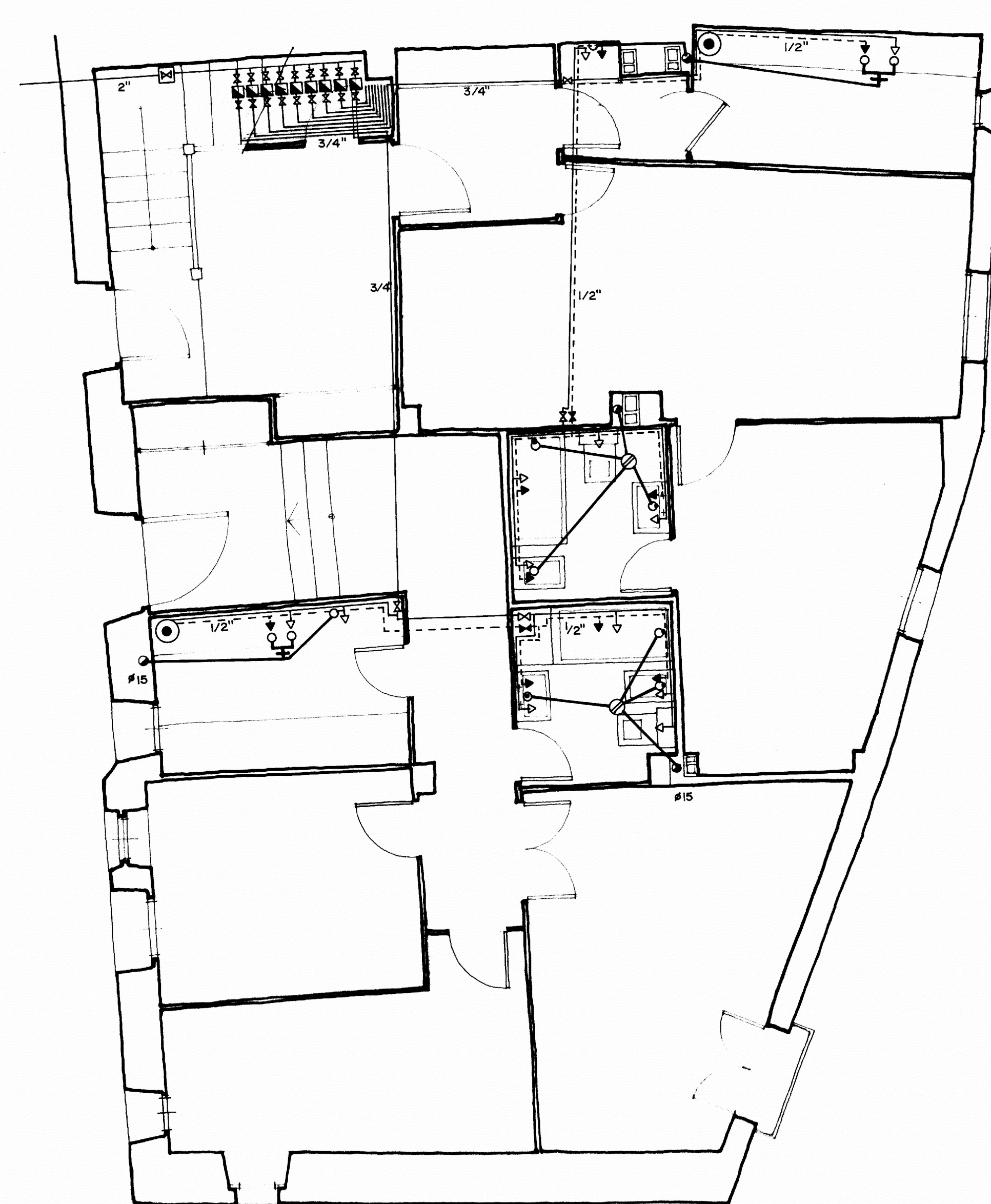
PLANTA 2
