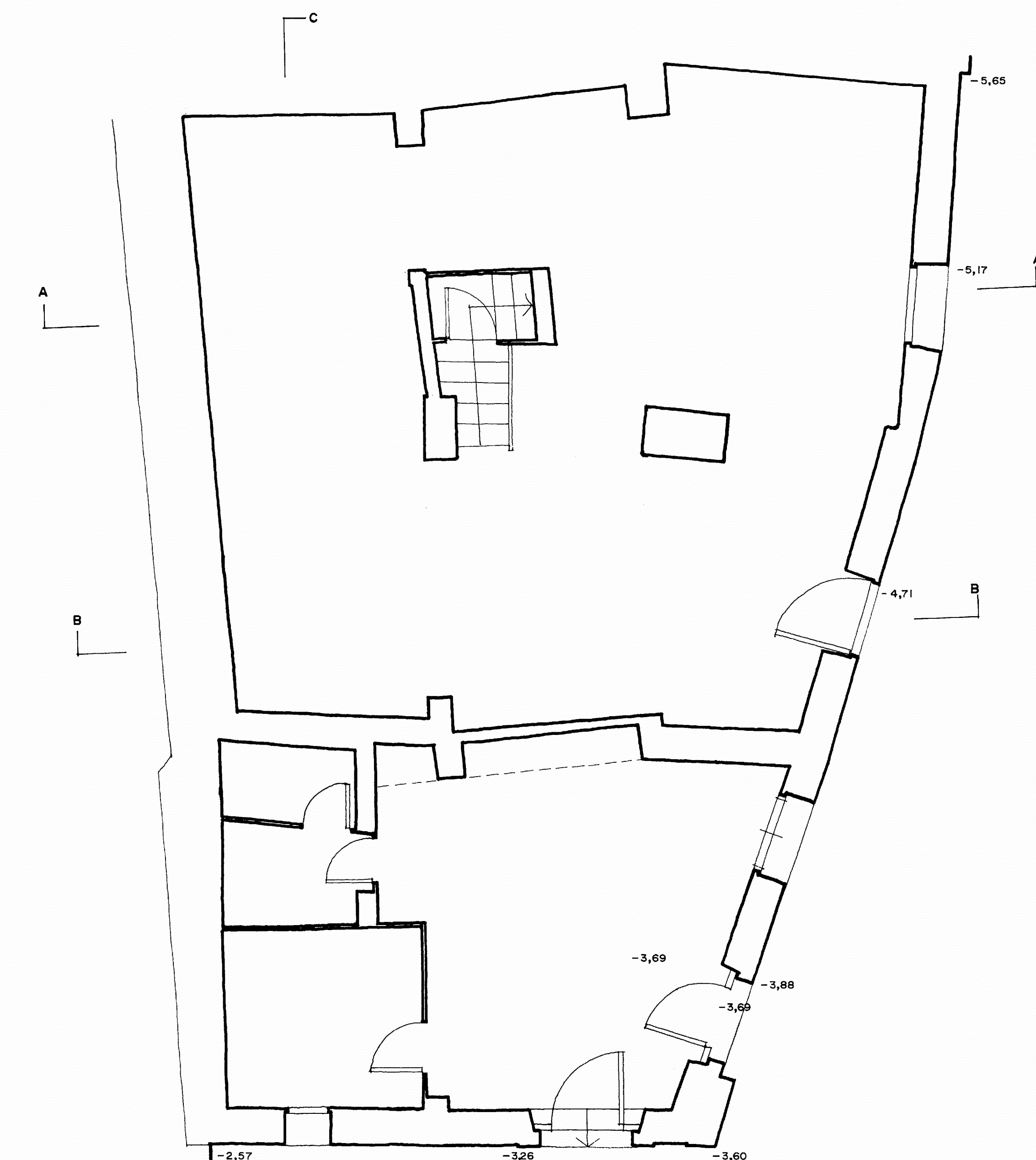
PLANTA 1
