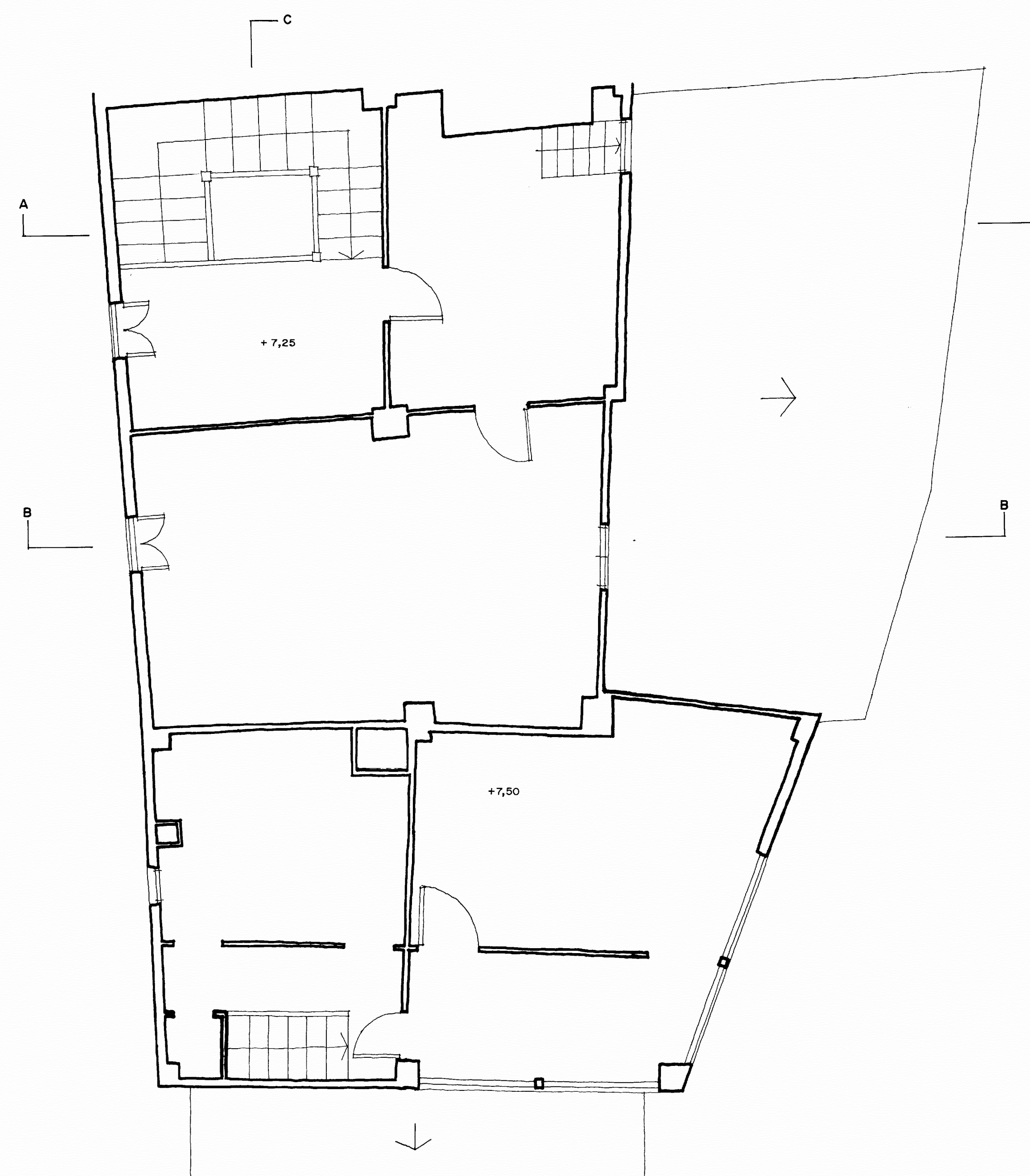
PLANTA 5
