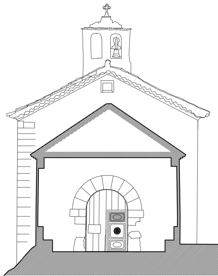
ALZADO NORTE
