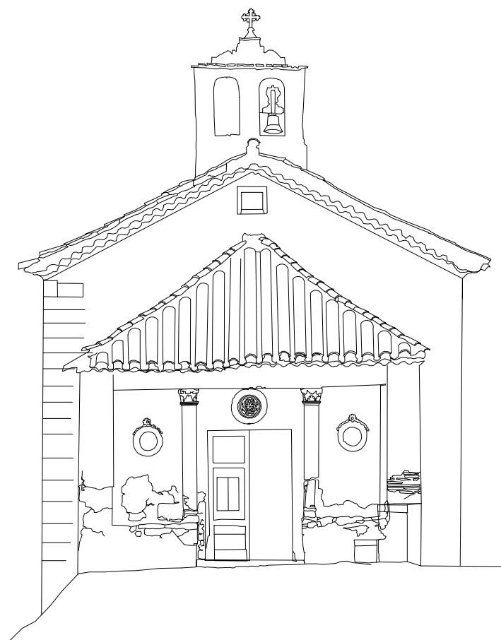
ALZADO NORTE
