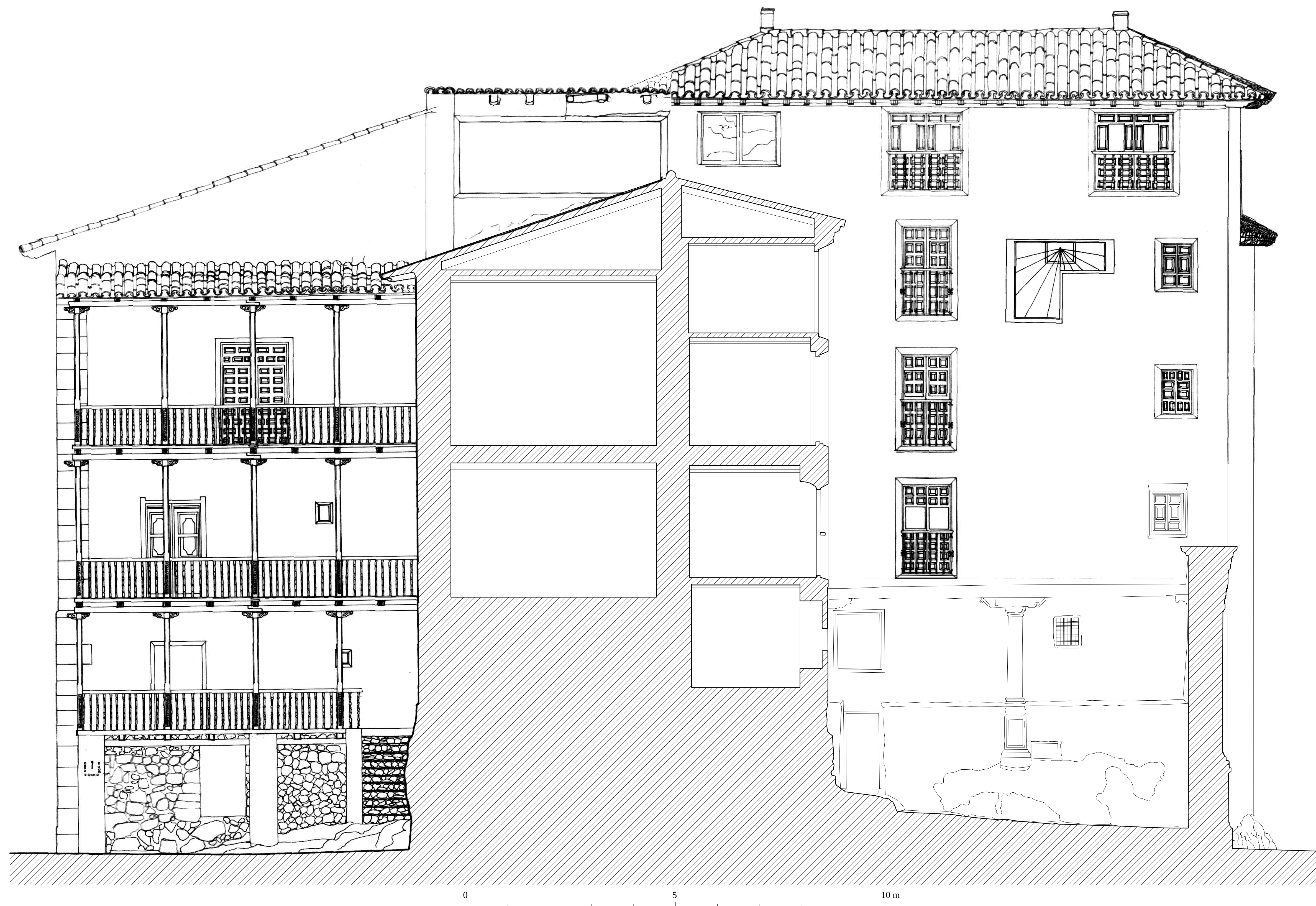
PALACIO EPISCOPAL DE ALBARRACIN. SECCION TRANSVERSAL
