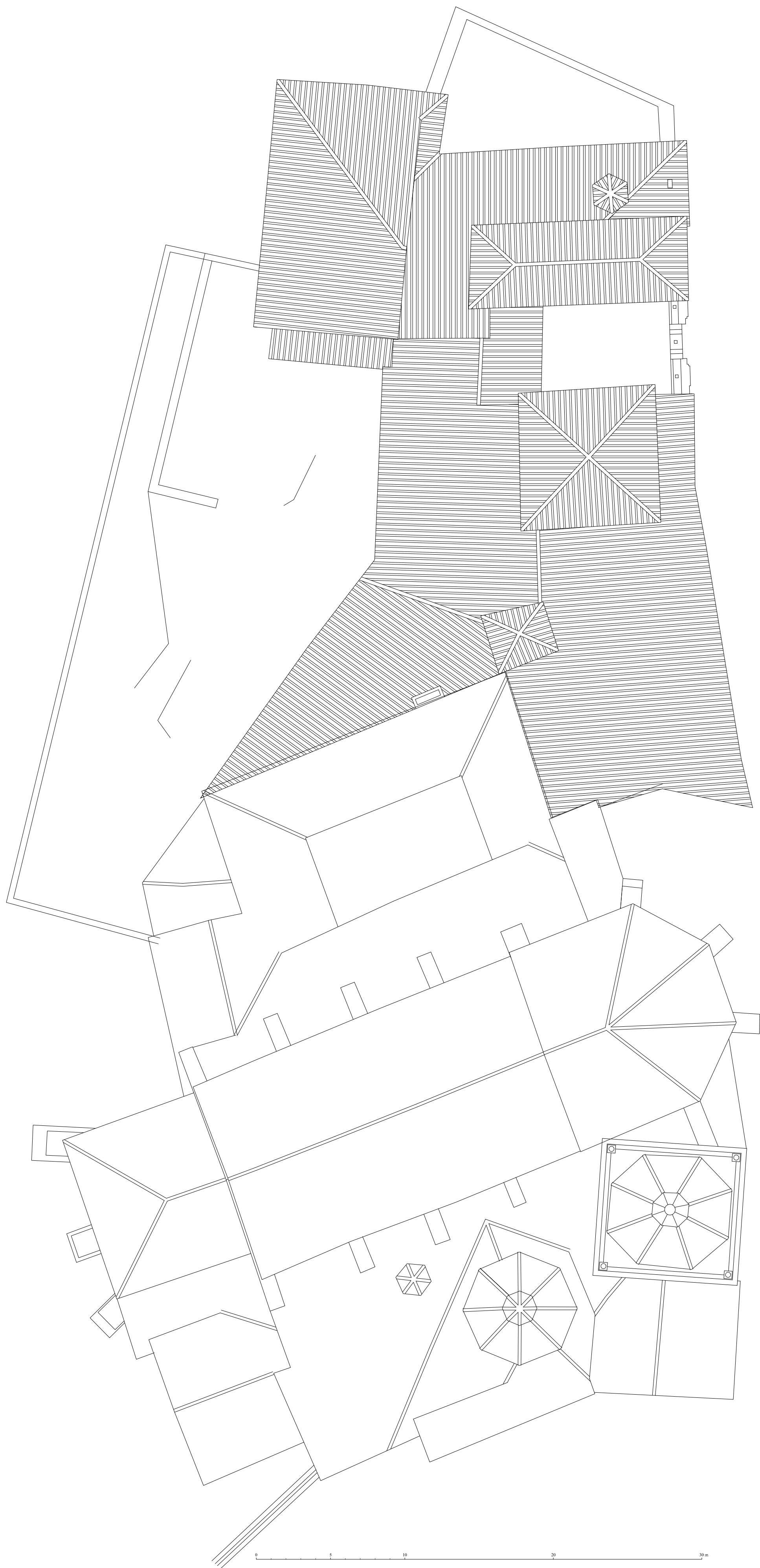
PALACIO EPISCOPAL DE ALBARRACIN. PLANTA DE CUBIERTAS
