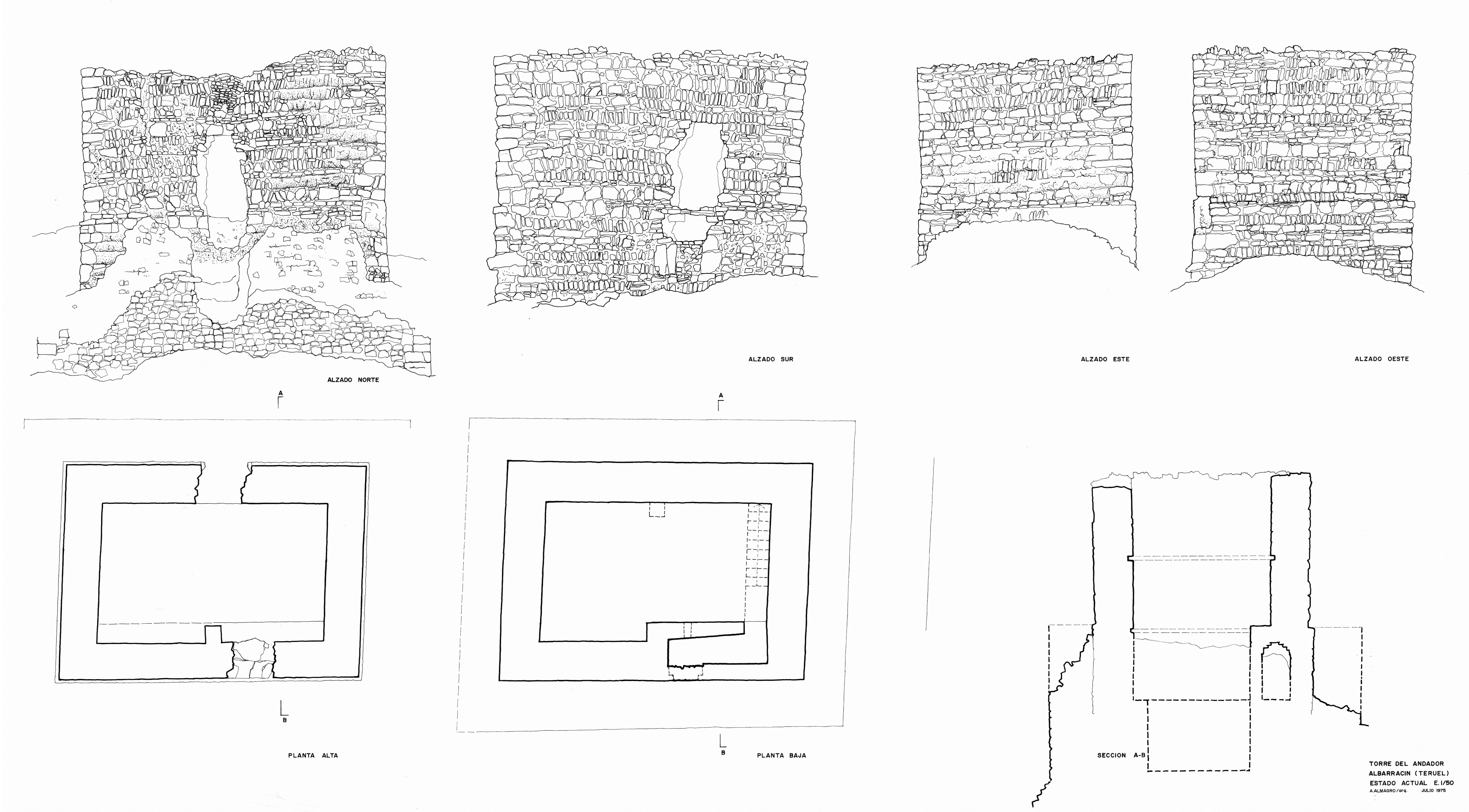
TORRE DEL ANDADOR. ALBARRACIN (TERUEL). ESTADO INICIAL
