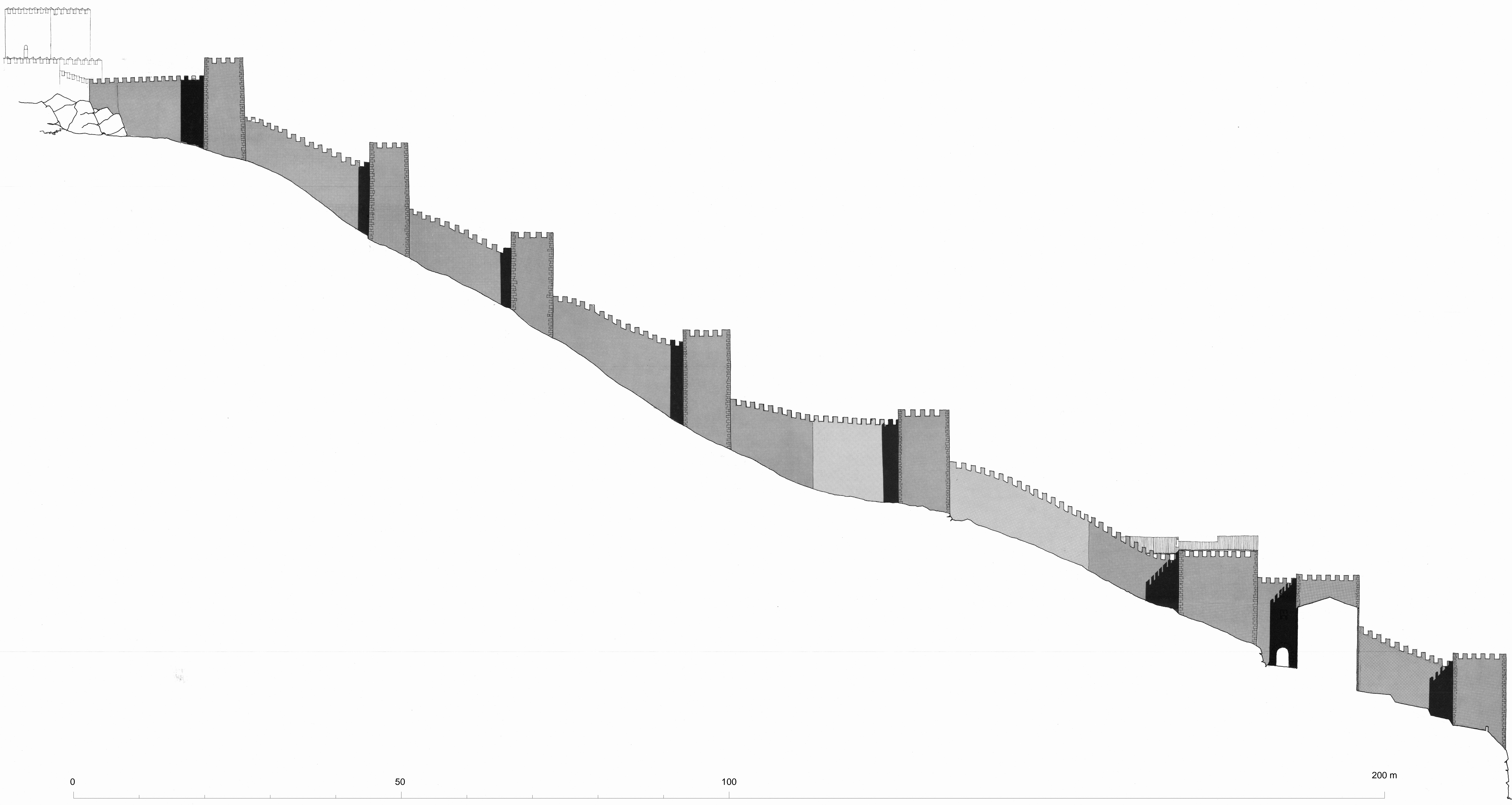
MURALLAS DE ALBARRACIN. RECINTO EXTERIOR. HIPOTESIS DEL ALZADO OESTE
