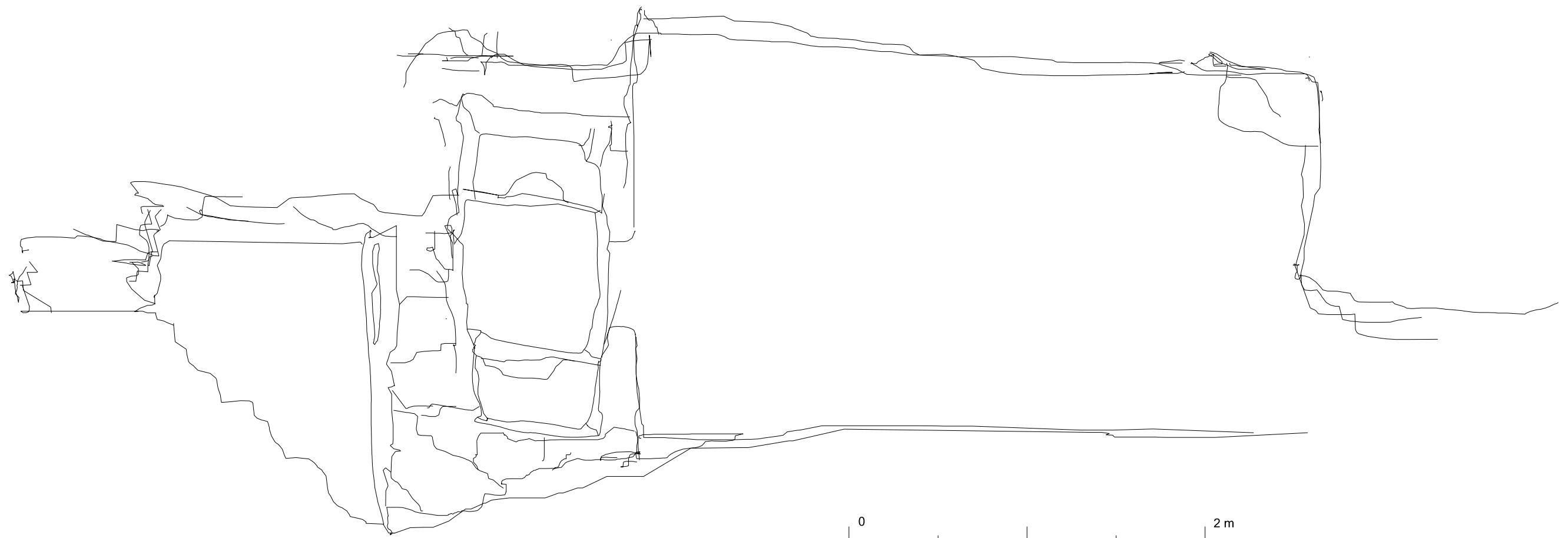
SAUNA DE ULACA ( Solosancho, Avila ) A. Almagro / arq. 1993
