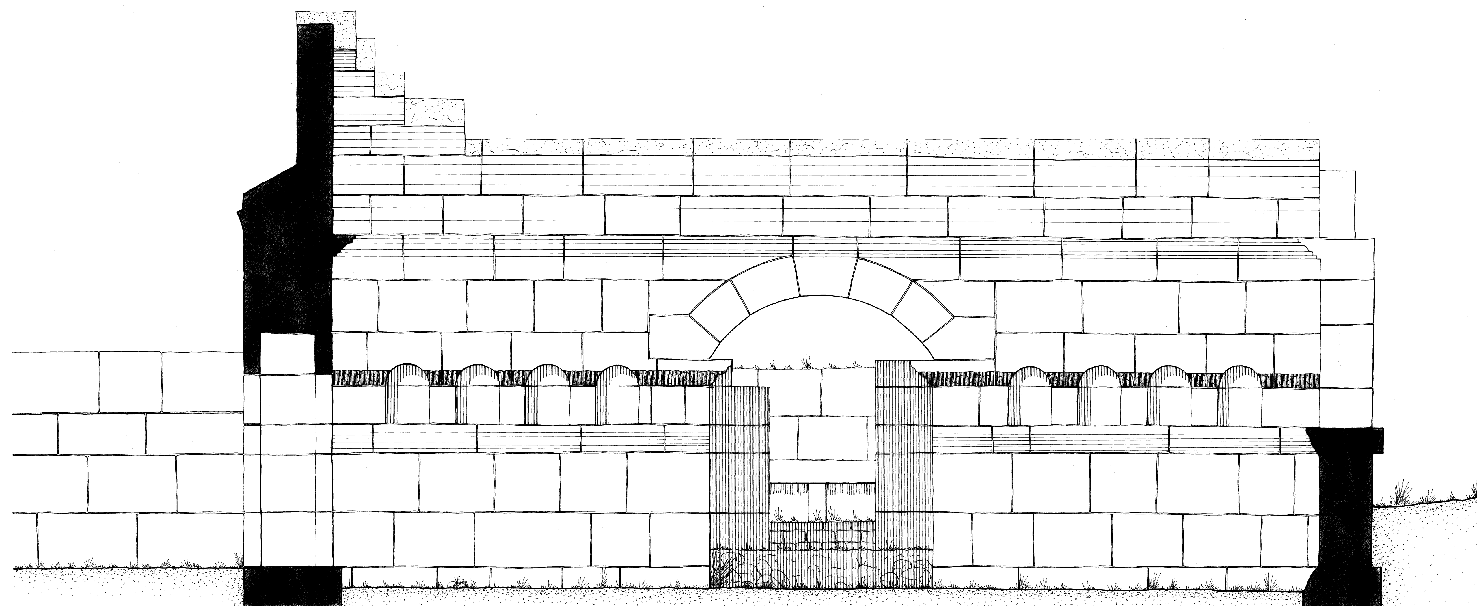
SECCION B-B
