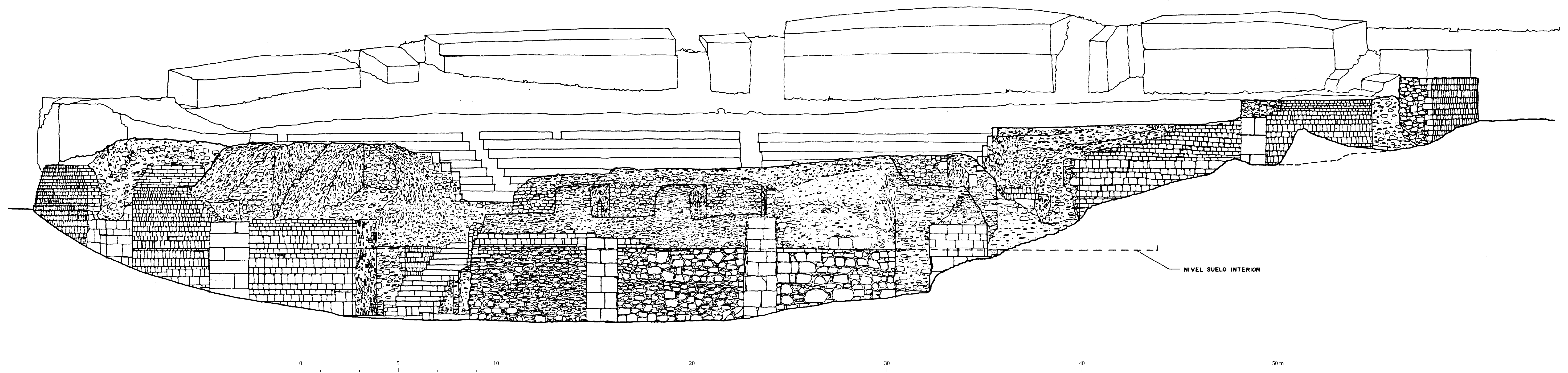
ANFITEATRO DE SEGOBRIGA (CUENCA). ALZADO NORTE. ESTADO INICIAL
