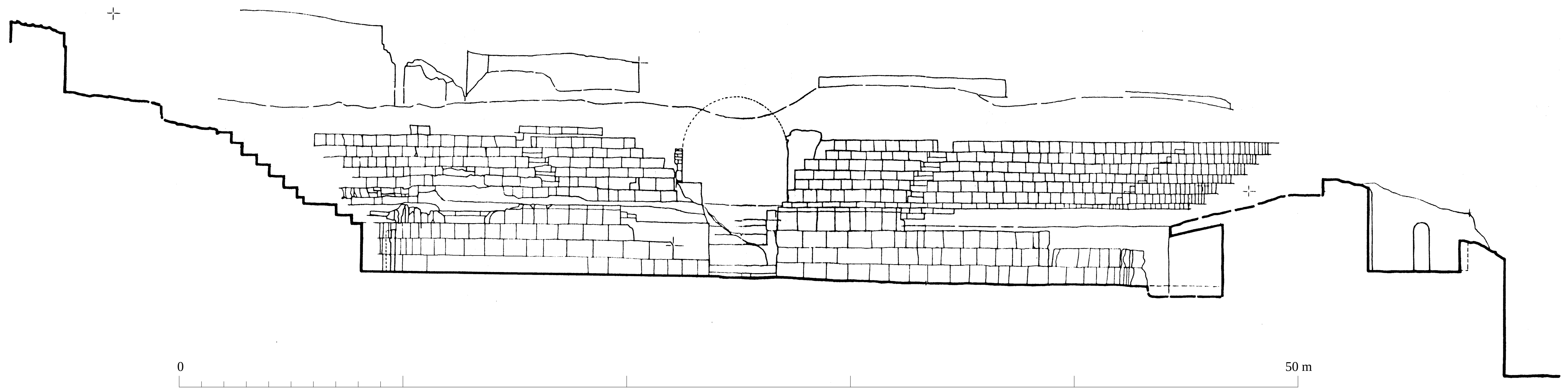
SECCION TRANSVERSAL DEL ANFITEATRO DE SEGOBRIGA (CUENCA)
