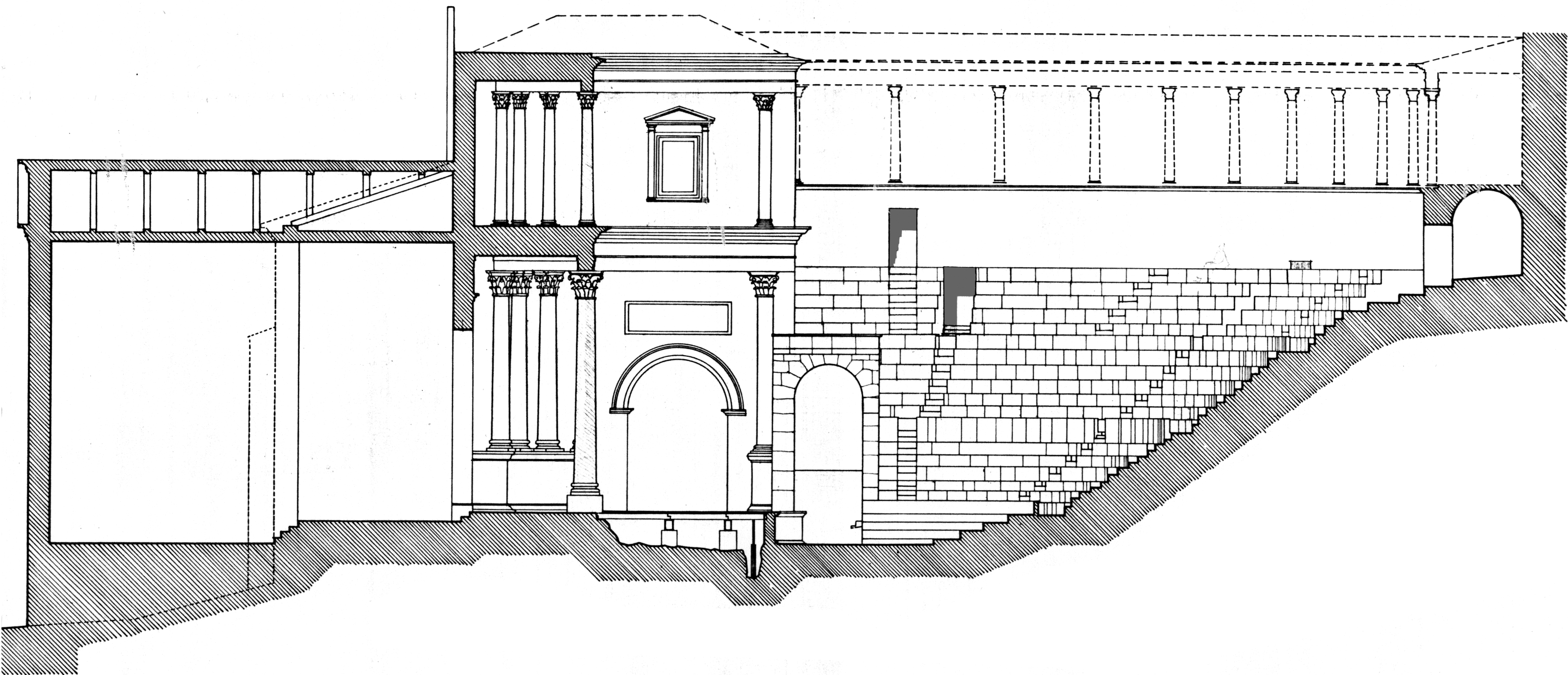
TEATRO ROMANO DE SEGOBRIGA SECCION (RECONSTRUCCION) E 1/100
